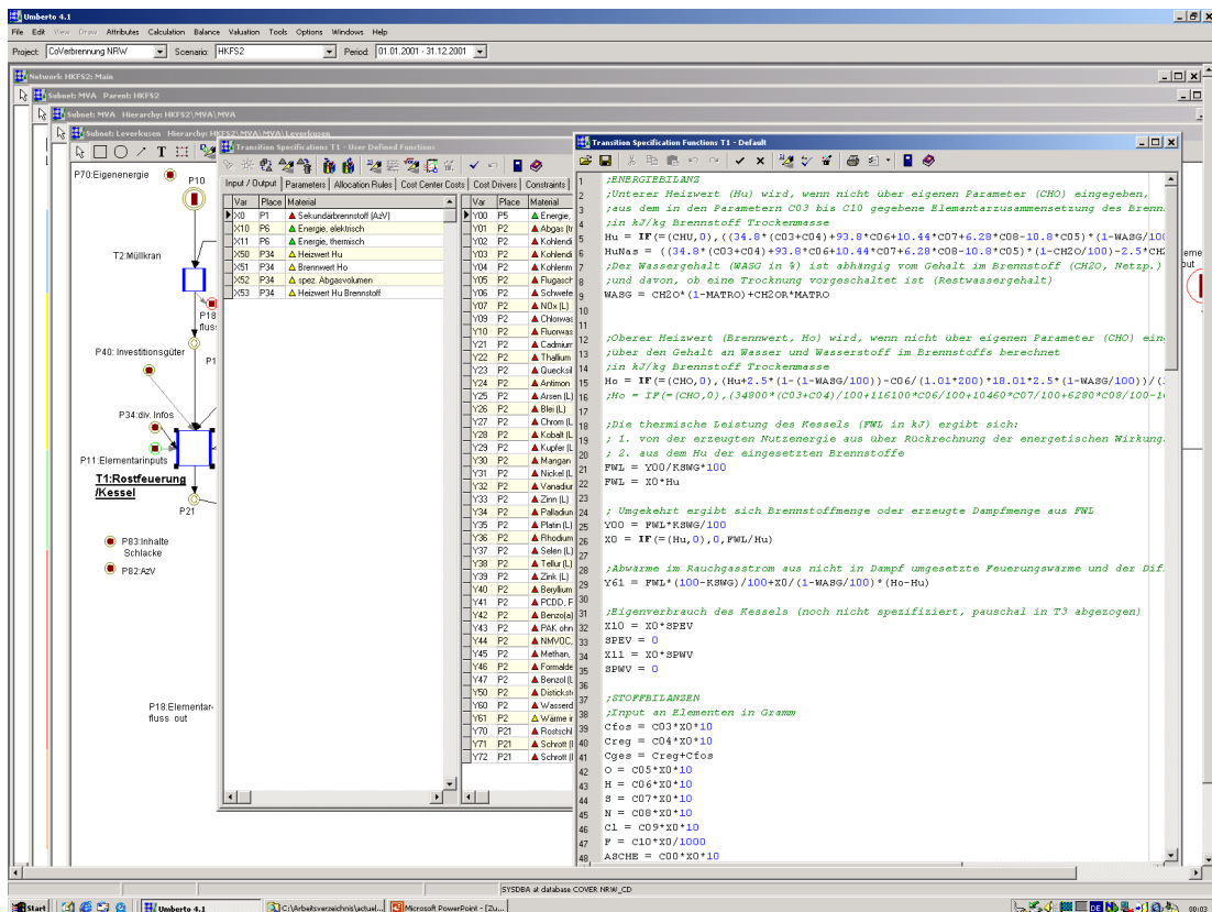
Abb. 3-3 Teilmodell einer Müllverbrennungsanlage sowie Rechenvorschriften für den Rostfeuerungskessel mit der Software Umberto®
