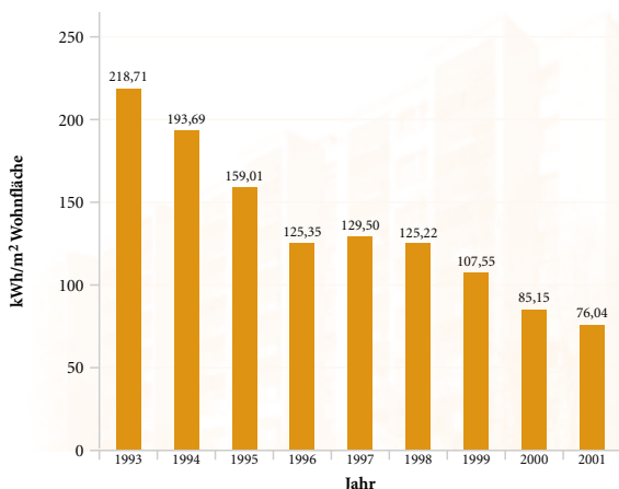
WGLi - Energieverbrauch eines Bautyps Entwicklung des Heizenergieverbrauchs in WBS 70/5
