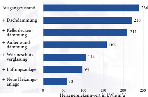
60er Jahre Mehrfamilienhaus – Energieeinsparung
