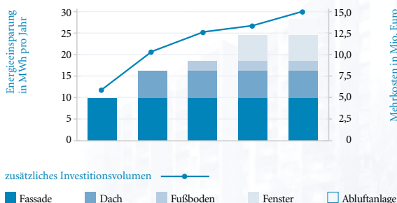
Einsparpotenzial durch Wärmedämmung im Gebäudebestand der Wohnungsunternehmen im GdW und zusätzliches Investitionsvolumen
