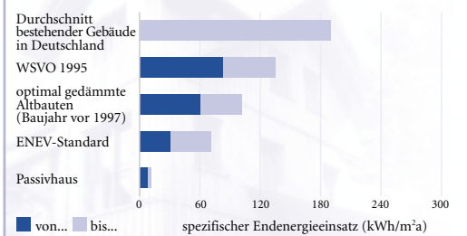
Spezifische Endenergiekennwerte verschiedener Baustandards
