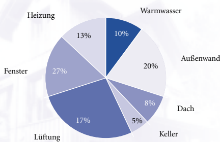
60er Jahre Mehrfamilienhaus – Wärmeverluste
