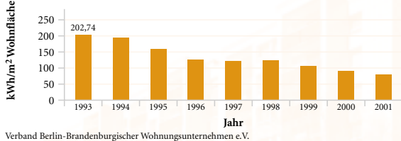
WGLi - Entwicklung des Heizenergieverbrauchs in mehr als 10.000 Wohnungen (Prefab Building) in Berlin
