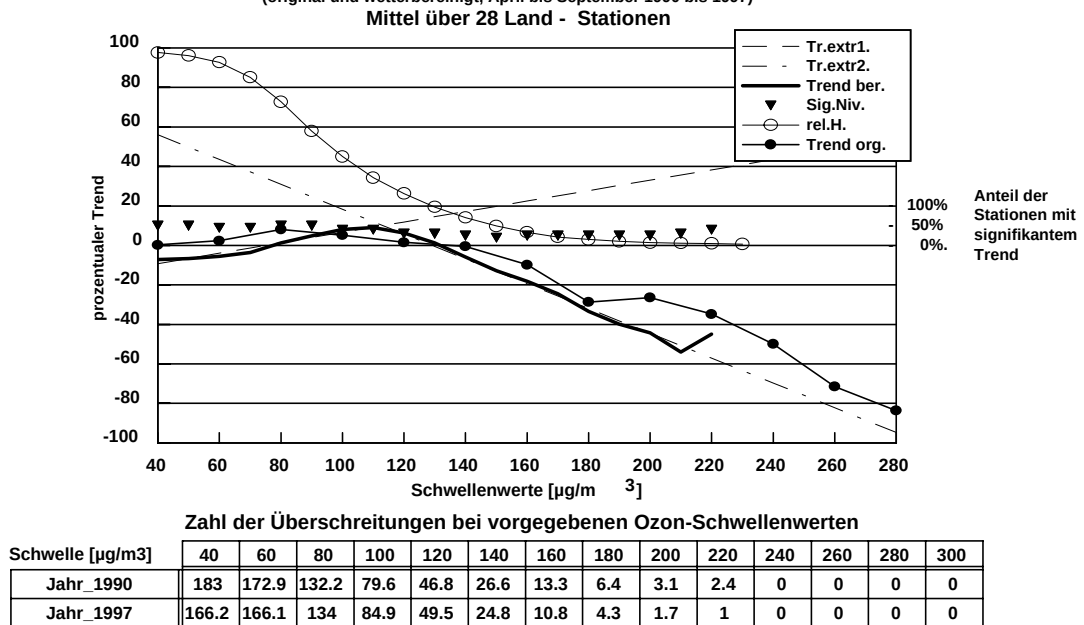
Abb. 24: Trend der Überschreitungshäufigkeit bei vorgegebenen Schwellenwerten (original und wetterbereinigt, April bis September 1990 bis 1997)
