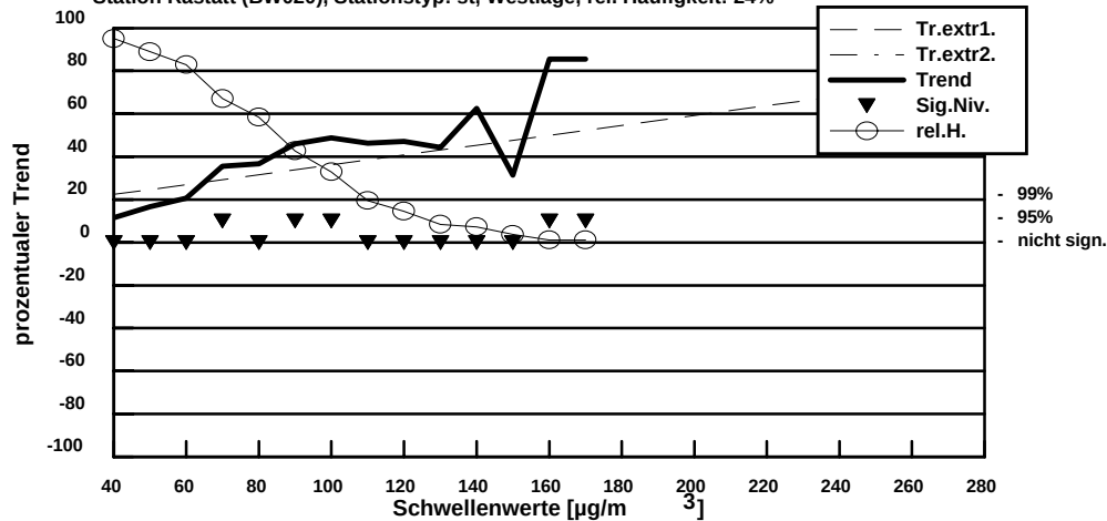
Abb. 28: Trend der Überschreitungshäufigkeit bei vorgegebenen Schwellenwerten (wetterbereinigt, April bis September 1990 bis 1997)
