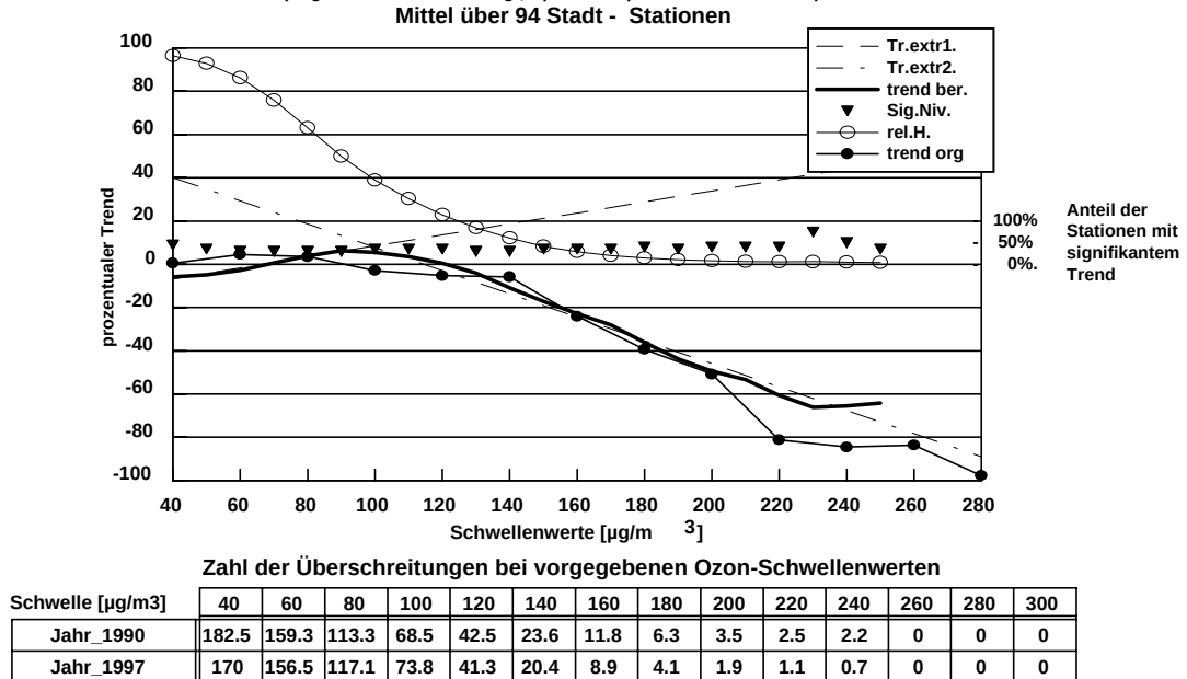
Abb. 23: Trend der Überschreitungshäufigkeit bei vorgegebenen Schwellenwerten (original und wetterbereinigt, April bis September 1990 bis 1997)
