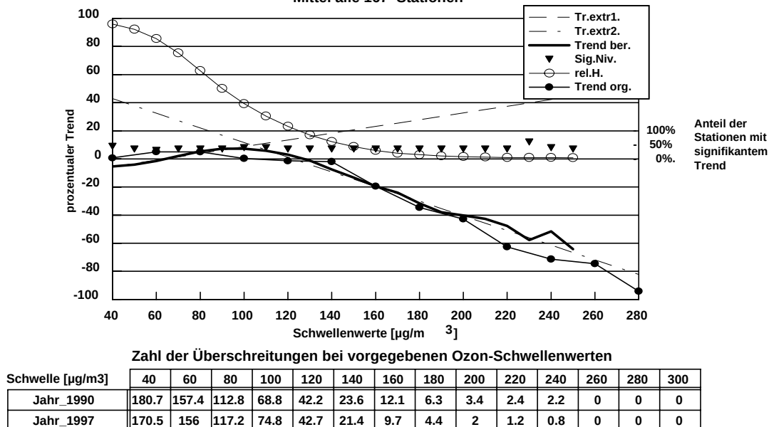
Abb. 26: Trend der Überschreitungshäufigkeit bei vorgegebenen Schwellenwerten (original und wetterbereinigt, April bis September 1990 bis 1997) Mittel alle 167 Stationen
