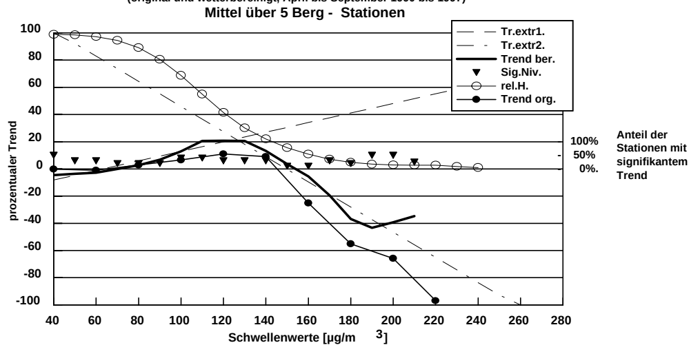
Zahl der Überschreitungen bei vorgegebenen Ozon-Schwellenwerten
