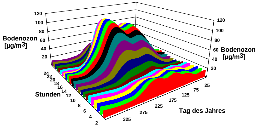
Abb. 4: Splineinterpolierter Jahresgang des Bodenozone
