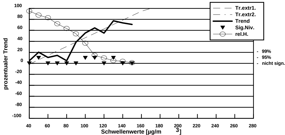
Abb. 27: Trend der Überschreitungshäufigkeit bei vorgegebenen Schwellenwerten (wetterbereinigt, April bis September 1990 bis 1997)
