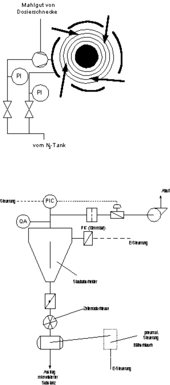
Abb. 6: Ausgewählte Funktionsgruppen des Miconizers
