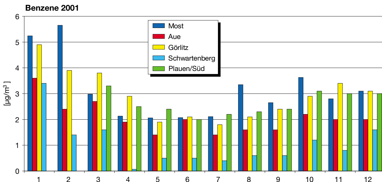
Figure 11. Monthly mean concentration in \mu\text{g}/\text{m}^3 of benzene in 2001 Obrázek 11. Měsíční průměrné koncentrace benzeny v \mu\text{g}/\text{m}^3 v roce 2001 Abbildung 11. Monats- und Jahresmittel der Benzolkonzentrationen 2001 [ \mu\text{g}/\text{m}^3 ] Rysunek 11. Średniomiesięczne stężenia benzeny w \mu\text{g}/\text{m}^3 w 2001 roku
