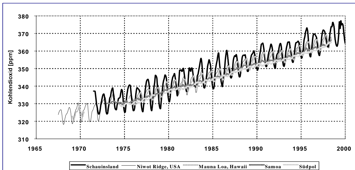
Abbildung 24: Langzeitrend der Monatsmittel der Kohlendioxidkonzentrationen vom Schauinsland im Vergleich zu Stationen auf Hawaii (Mauna Loa), in Niwot Ridge (USA), in Samoa und am Südpol zwischen 1968 bis 2000
