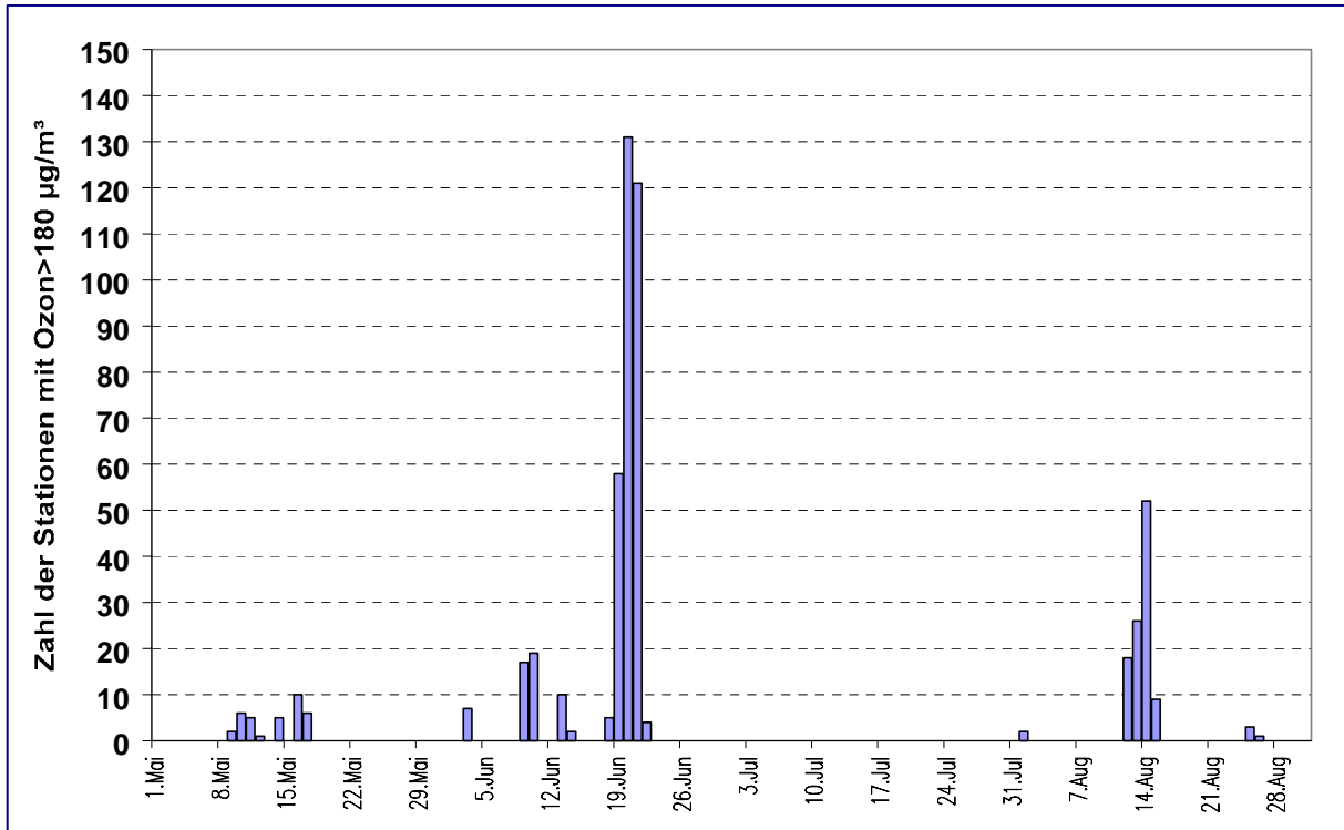
Abbildung 49: Zahl der Tage und Stationen mit Überschreitungen von 180 \mu\text{g}/\text{m}^3 (Stundenmittel)
