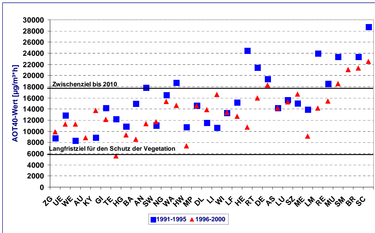
Abbildung 15: AOT40-Werte zum Schutz der Vegetation an allen Messstellen des UBA
