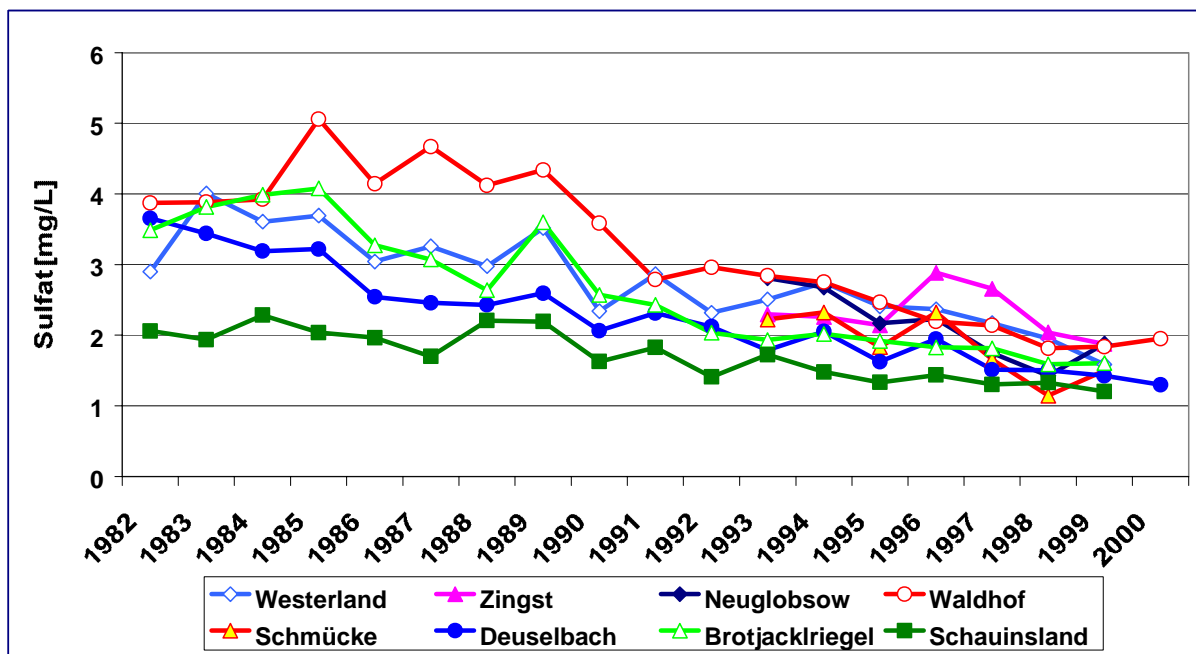
Abbildung 33: Jahresmittel SO_4^- -Ionen-Konzentration (seesalzkorrigiert) im Niederschlag von 1982 bis 2000 für die personell besetzten UBA-Messstellen.
