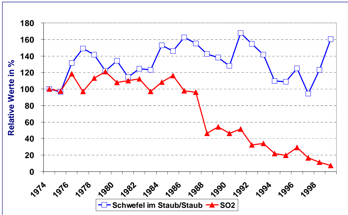
Abbildung 30: Massen-Verhältnis Schwefel im Schwebstaub/Gesamtstaub und SO_2 -Konzentrationen der Jahresmittel zwischen 1974 und 1999, im Mittel über 4 Messstellen (Waldhof, Deuselbach, Schauinsland und Brotjacklriegel) in den alten Bundesländern (ohne Westerland wegen des hohen Seesalzanteils), normiert auf das Jahr 1974
