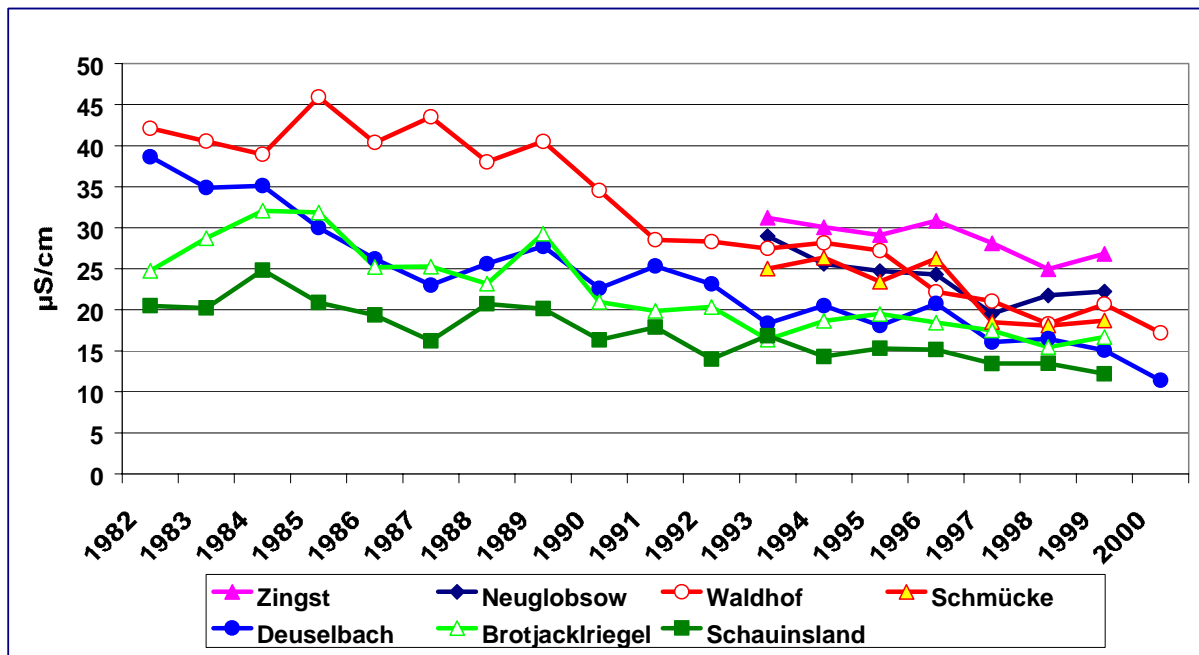
Abbildung 35: Jahresmittel der Leitfähigkeit des Niederschlags von 1982 bis 2000 für die personell besetzten UBA-Messstellen.
