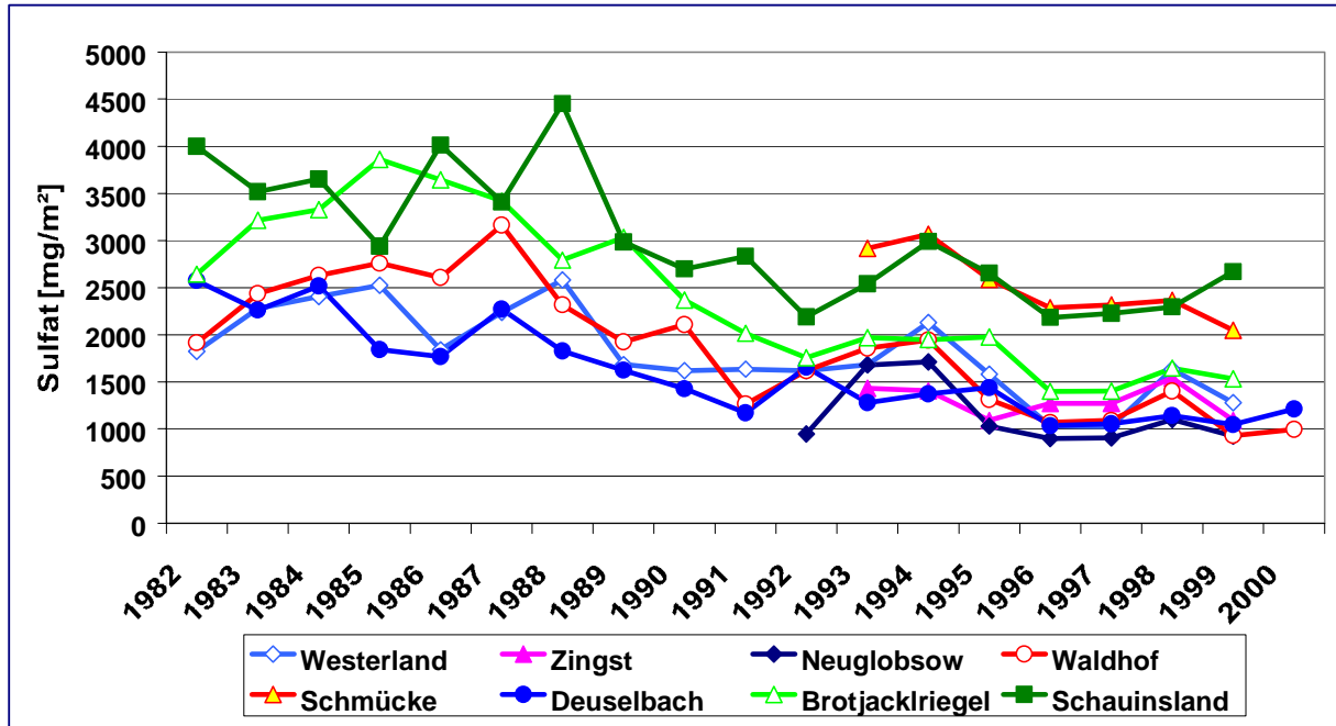
Abbildung 37: Jährliche Depositionen von SO_4^{2-} (seesalzkorrigiert) an den Messstellen des UBA zwischen 1982 bis 2000.
