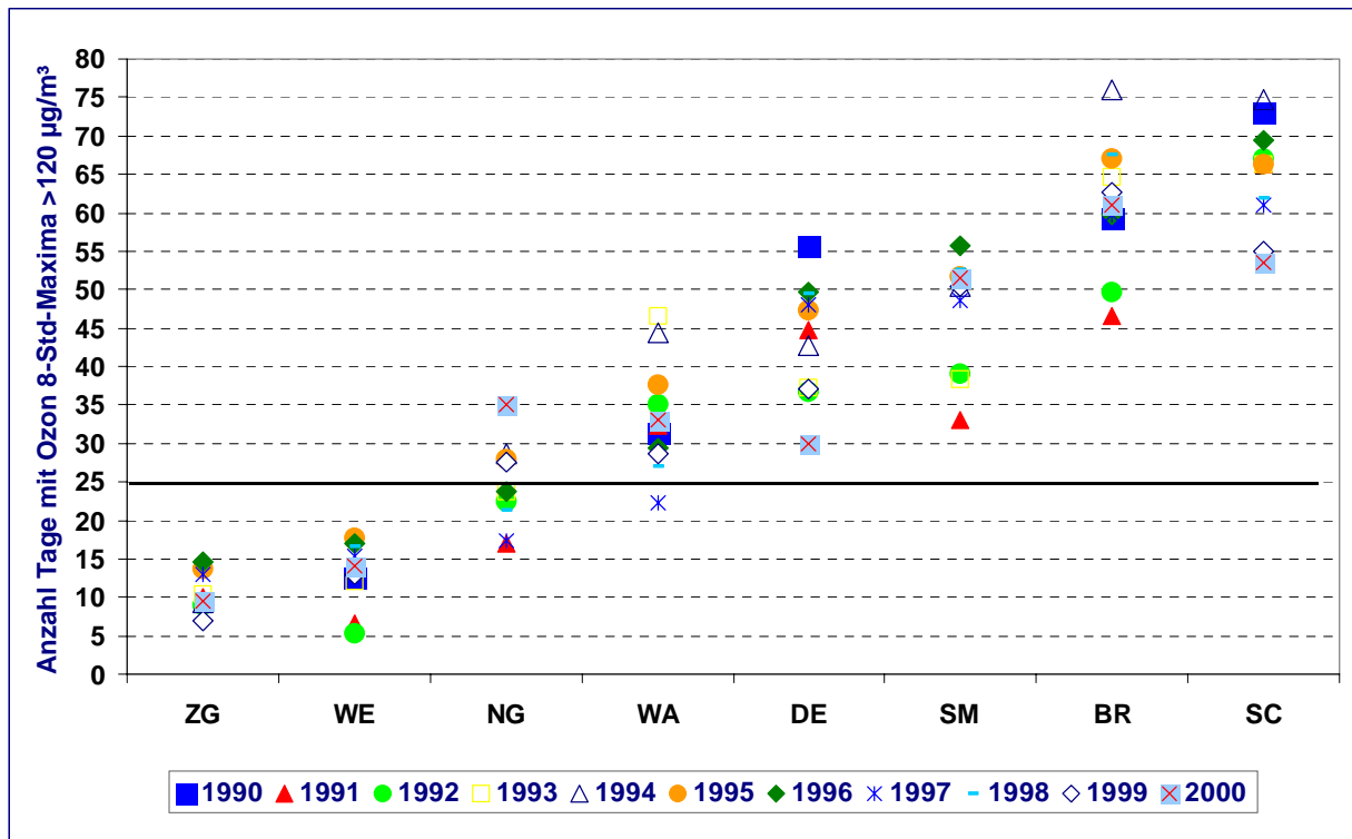
Abbildung 13: Anzahl der Tage/Jahr mit Überschreitungen von gleitenden 8-h-Mitteln > 120 µg/m³ Ozon an den 8 personell besetzten Messstellen des Umweltbundesamts es zwischen 1990 und 2000, nach Stationshöhe sortiert.
