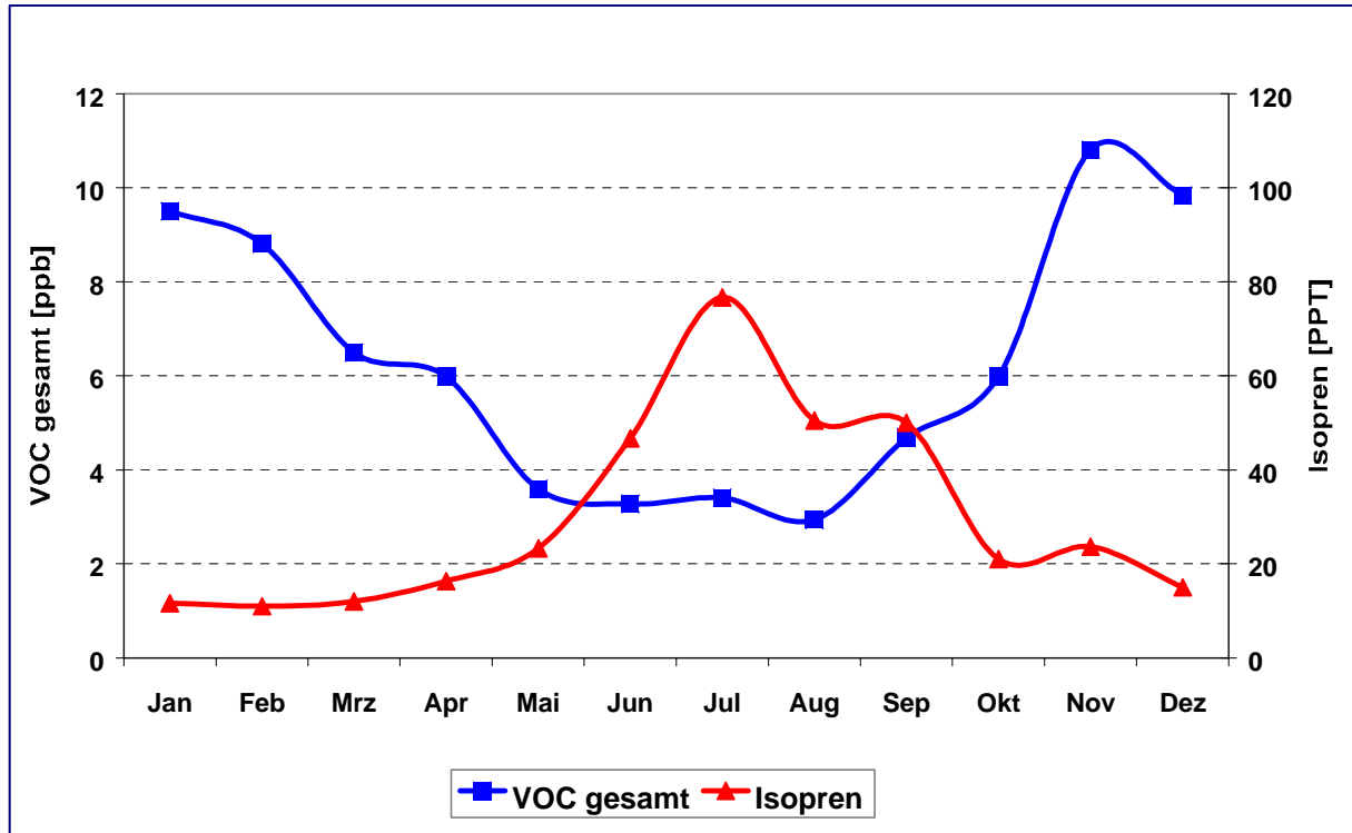
Abbildung 20: Mittlerer Jahrgang von VOC gesamt und Isopren in Waldhof für 1998-2000.
