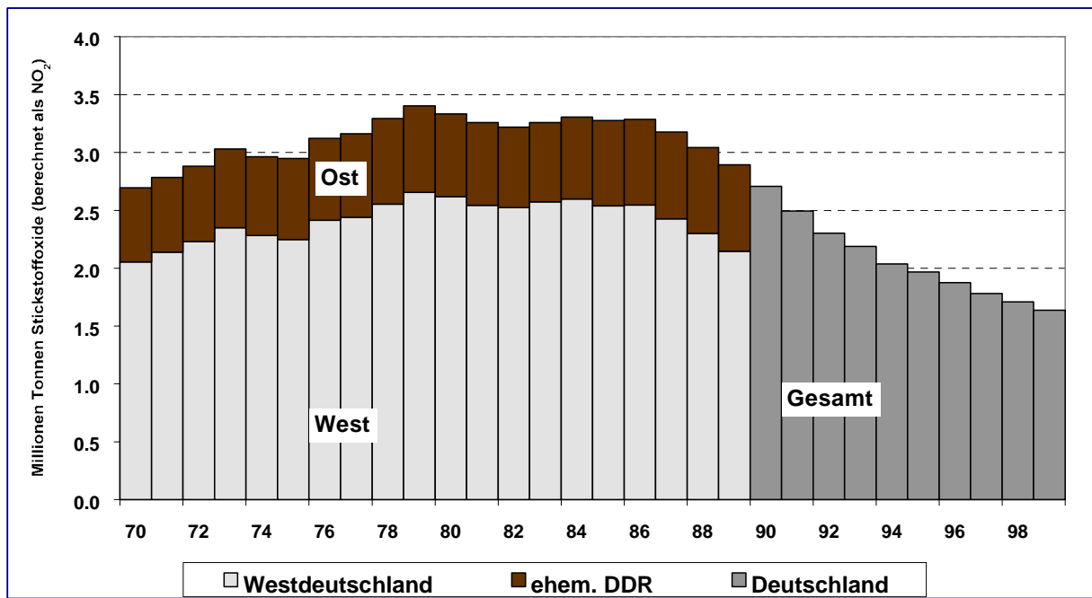
Abbildung 11: Jährliche Stickstoffdioxid-Emissionen (berechnet als \text{NO}_2 ) in Deutschland von 1970 bis 1999 (Ref. 1)
