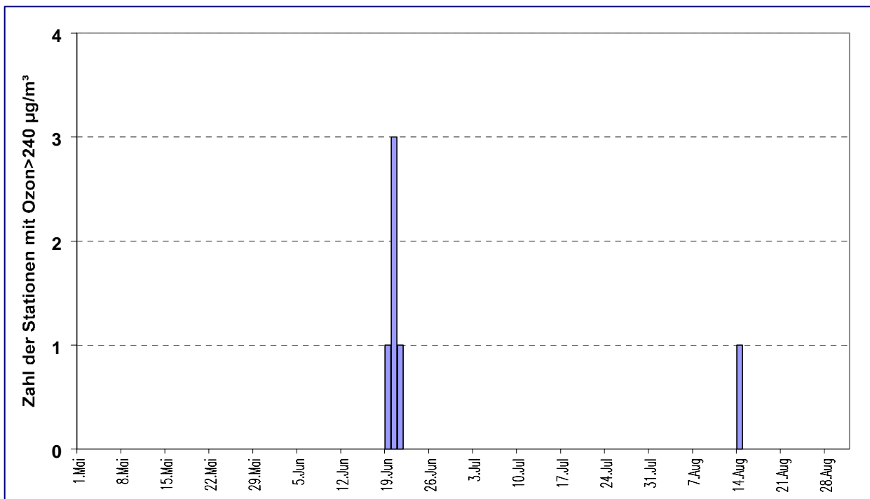
Abbildung 50: Zahl der Tage und Stationen mit Überschreitungen von 240 \mu\text{g}/\text{m}^3 (Stundenmittel)
