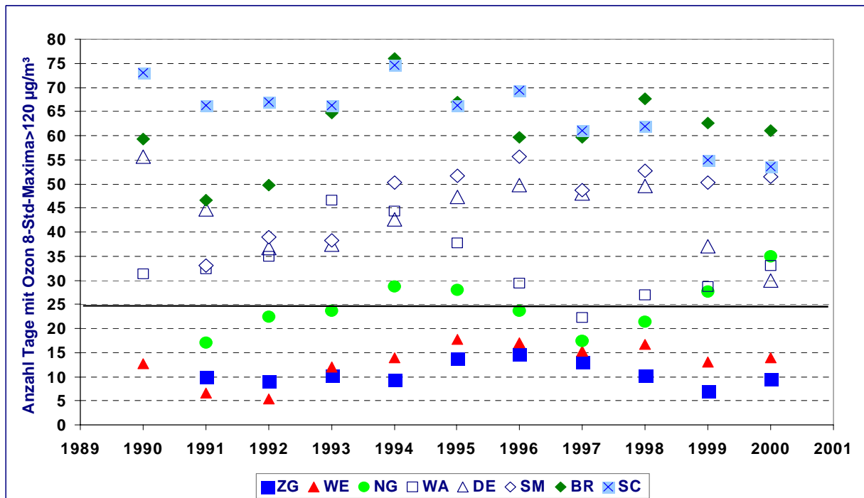
Abbildung 14: Anzahl der Tage/Jahr mit Überschreitungen von gleitenden 8-h-Mitteln > 120 µg/m³ Ozon an den 8 personell besetzten Messstellen des Umweltbundesamts es zwischen 1990 und 2000, nach Jahren sortiert.
