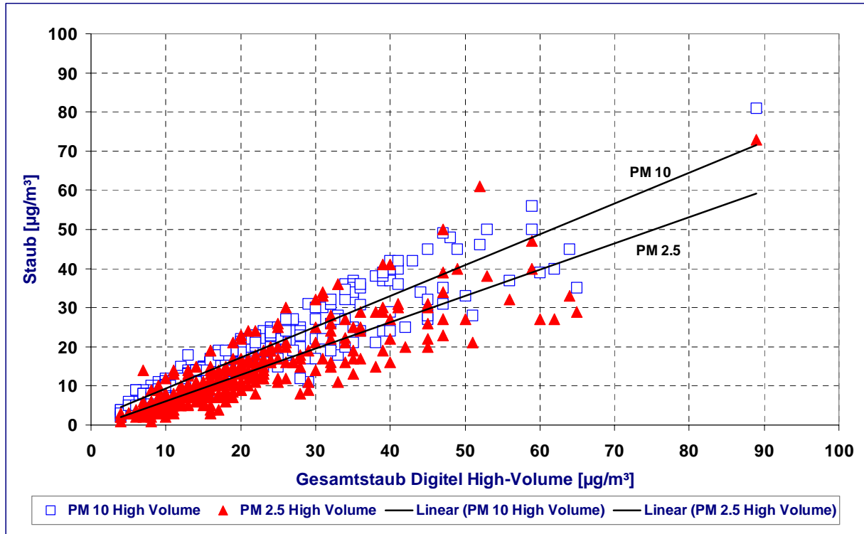
Abbildung 27: Vergleich von Staubmessungen in Waldhof in 2000 zwischen Gesamtstaub, PM_{10} und PM_{2.5}
