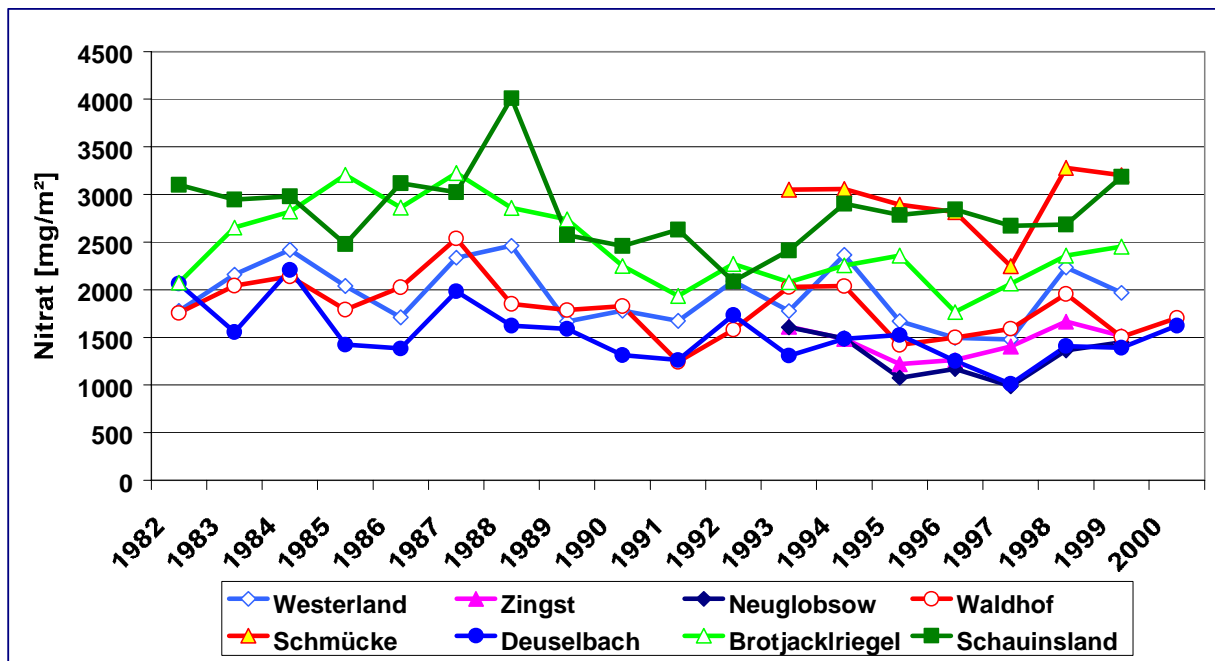
Abbildung 38: Jährliche Depositionen von NO_3^- an den Messstellen des UBA zwischen 1982 bis 2000.
