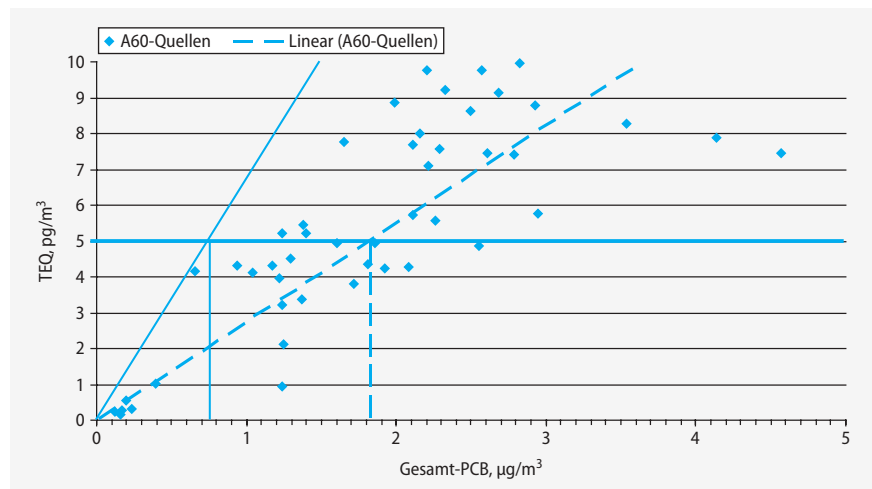
Abb. 3 ▲ PCB-TEQ-Werte in Abhängigkeit von PCB-Gesamtkonzentrationen in der Innenraumluft (UFOPLAN-Studie und BW-Plus-Studie), wenn Clophen-A60-Quellen (PCB-haltige Deckenplatten und Farbanstriche) vorliegen
