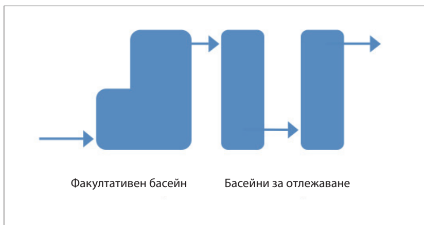
Фигура 2: Схематична хоризонтална проекция на система от стабилизационни басейни
