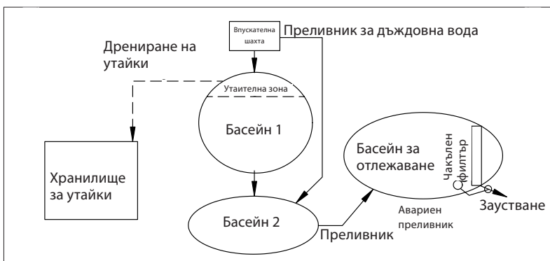
Фигура 7: Схема на система от естествени басейни в Съорен, Германия
