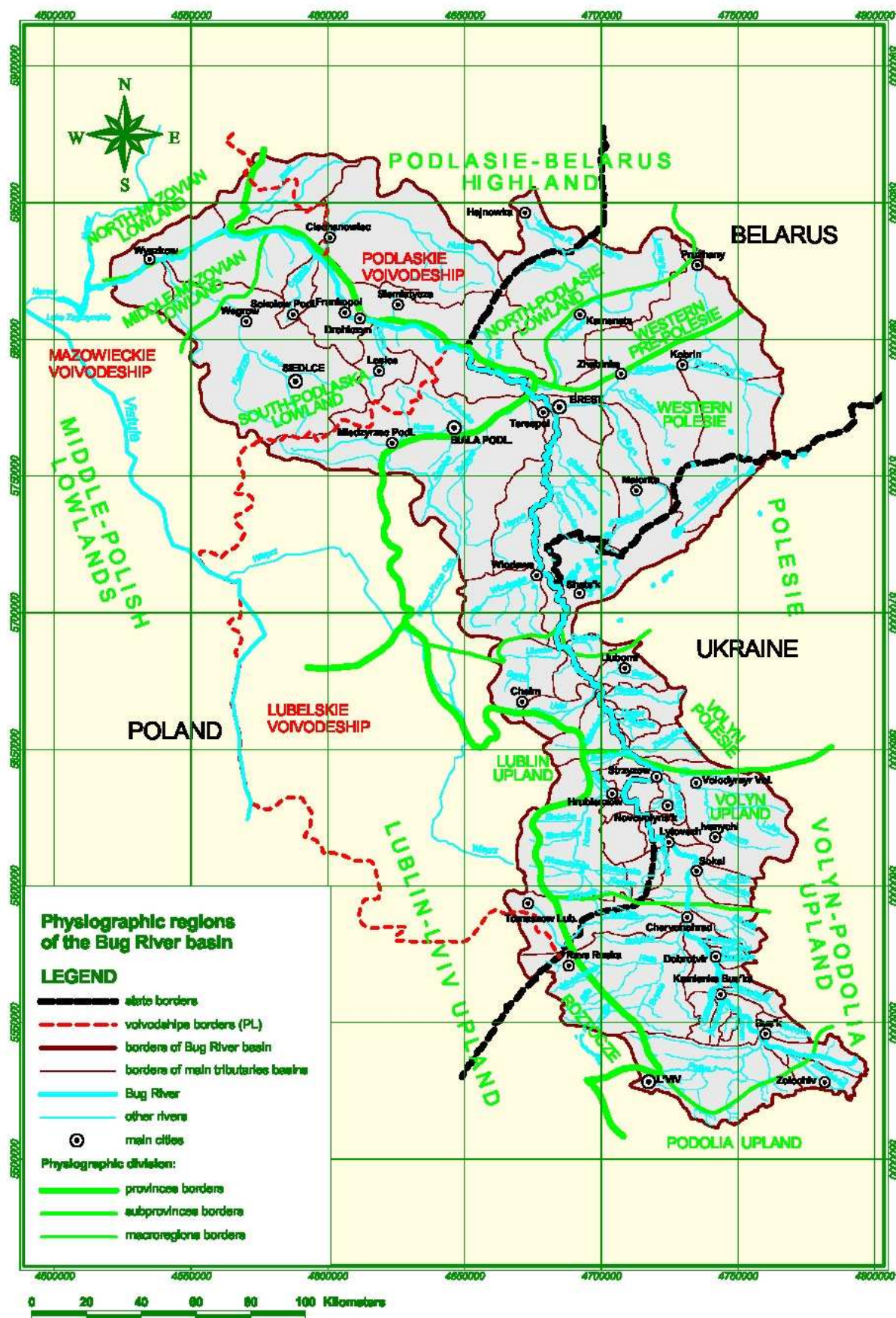
Малюнок 3: Фізіографічні регіони басейну ріки Західний Буг
