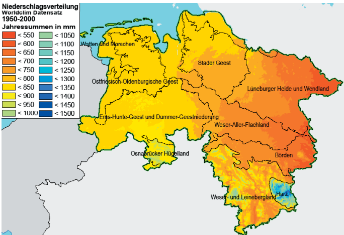
Abb. 2: Rezente durchschnittliche Jahresniederschlagssummen (Daten: WorldClim)
