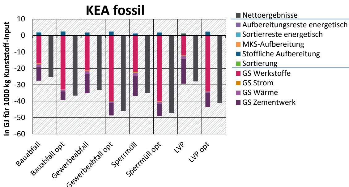
Abbildung 41: Die Verwertung von Kunststoffen unter dem Aspekt KEA (fos)
