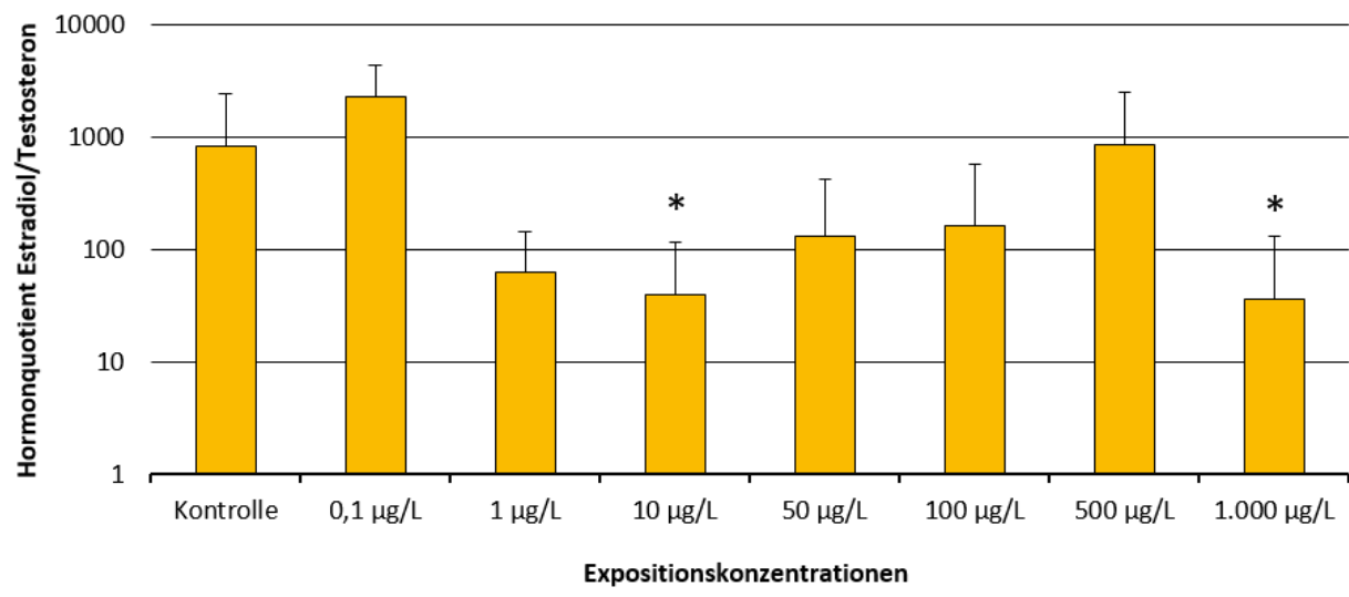
Abbildung 37: Hormonquotienten bei weiblichen Regenbogenforellen (Teilversuch Nr. 2, Metformin)
