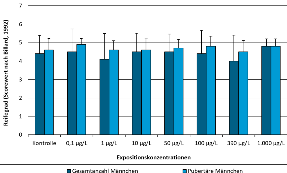
Abbildung 24: Reifegrade der Hoden (Teilversuch Nr. 1, Guanylurea)
