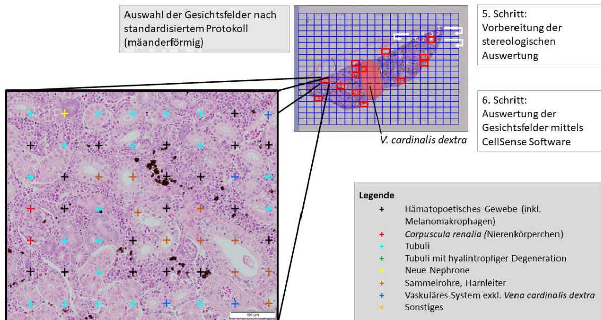
Abbildung 13: Schätzung der Volumendichte ( V_V ) der verschiedenen Nierenzelltypen
