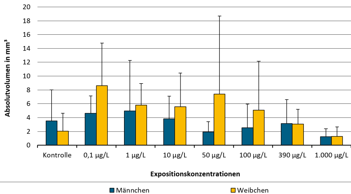
Abbildung 27: Absolutvolumina (V) neuer Nephronen subadulter Regenbogenforellen (Teilversuch Nr. 1, Guanylurea)
