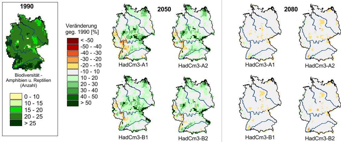
Abb. 4.4-4: Relative Veränderung in der Artenzahl von Amphibien und Reptilien gegenüber 1990. Datengrundlage ist eine Auswahl von 108 ausgewählten Amphibien und Reptilienarten mit europäischem Verbreitungsgebiet. Im Gegensatz zu anderen ATEAM-Ergebnissen liegen hier nur Szenarien für die mit dem GCM HadCM3 gerechneten Klimaszenarien vor.
