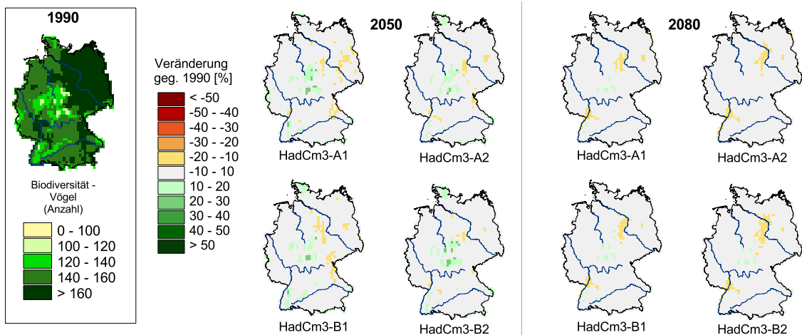
Abb. 4.4-5: Relative Veränderung in der Artenzahl von Vogelarten gegenüber 1990. Datengrundlage ist eine Auswahl von 383 ausgewählten Vogelarten mit europäischem Verbreitungsgebiet. Im Gegensatz zu anderen ATEAM-Ergebnissen liegen hier nur Szenarien für die mit dem GCM HadCM3 gerechneten Klimaszenarien vor.
