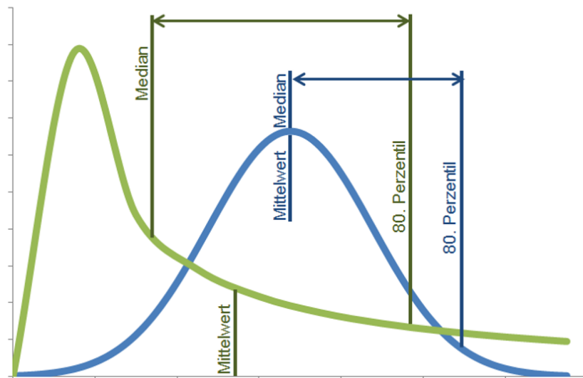
Abbildung 22: Skizze zu Lageparametern bei normal- und lognormal verteilten Analysenwerten
