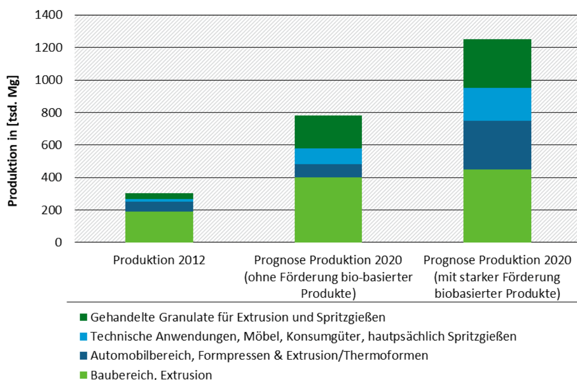
Abbildung 18: Prognose zur Produktion von Holz-Polymer-Verbundstoffen in Europa 195
