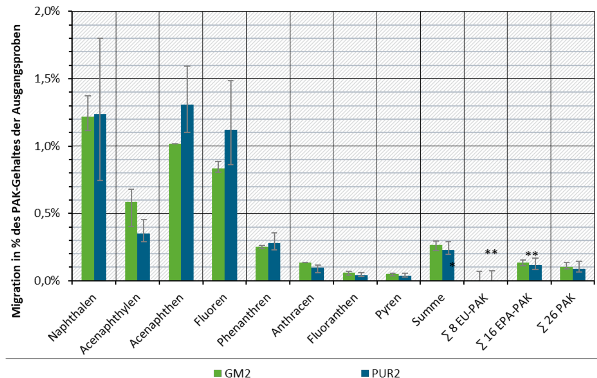
Abbildung 30 Relative Migrationrate der PAK aus Werkstoffproben mit Altreifenrezyklat nach JRC-Methode bezogen auf deren Gesamtgehalt in den Proben
