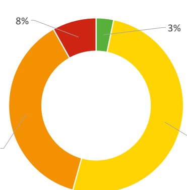
Abbildung: Ökologischer Zustand der Mittelgebirgsflüsse in Deutschland 2021
