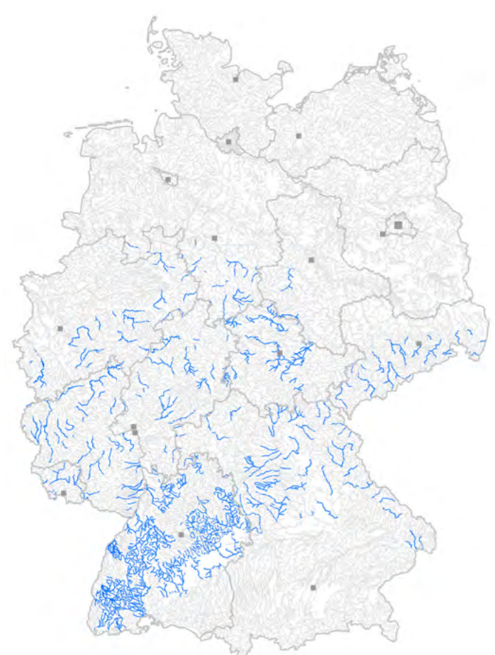
Vorkommen der Mittelgebirgsflüsse in Deutschland 2021; Details über interaktive Karte abrufbar: http://gis.uba.de/website/apps/gd/
