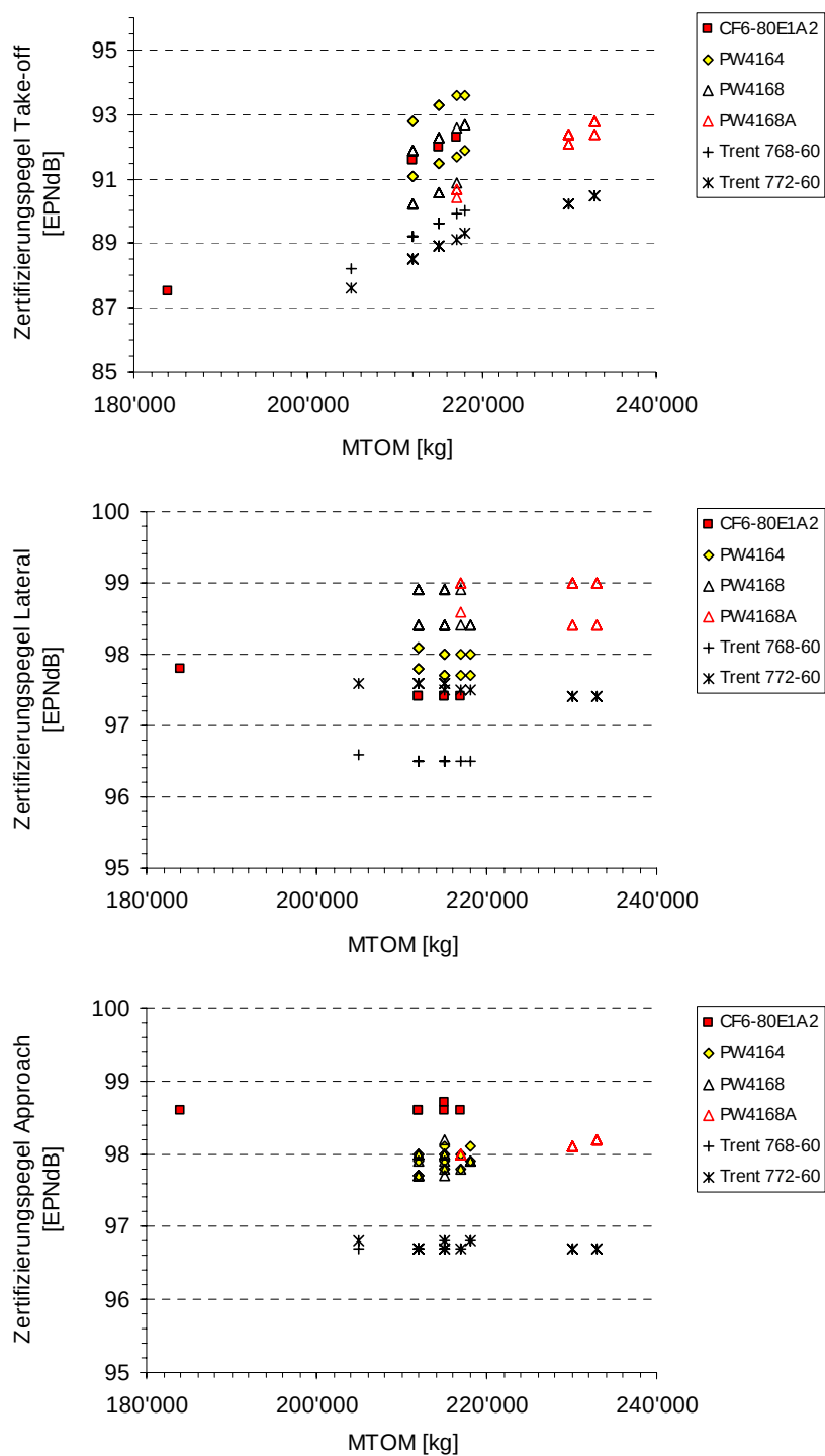
Abbildung 19 Zertifizierungspegel für unterschiedliche Konfigurationen für Airbus A 330-300
