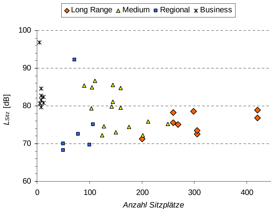
Abbildung 15 Ereignispegel L_{AE} (a) und sitzplatzbezogener Ereignispegel L_{Sitz} (b) für unterschiedliche Flugzeugkategorien in Abhängigkeit von der Sitzplatzzahl Starts
