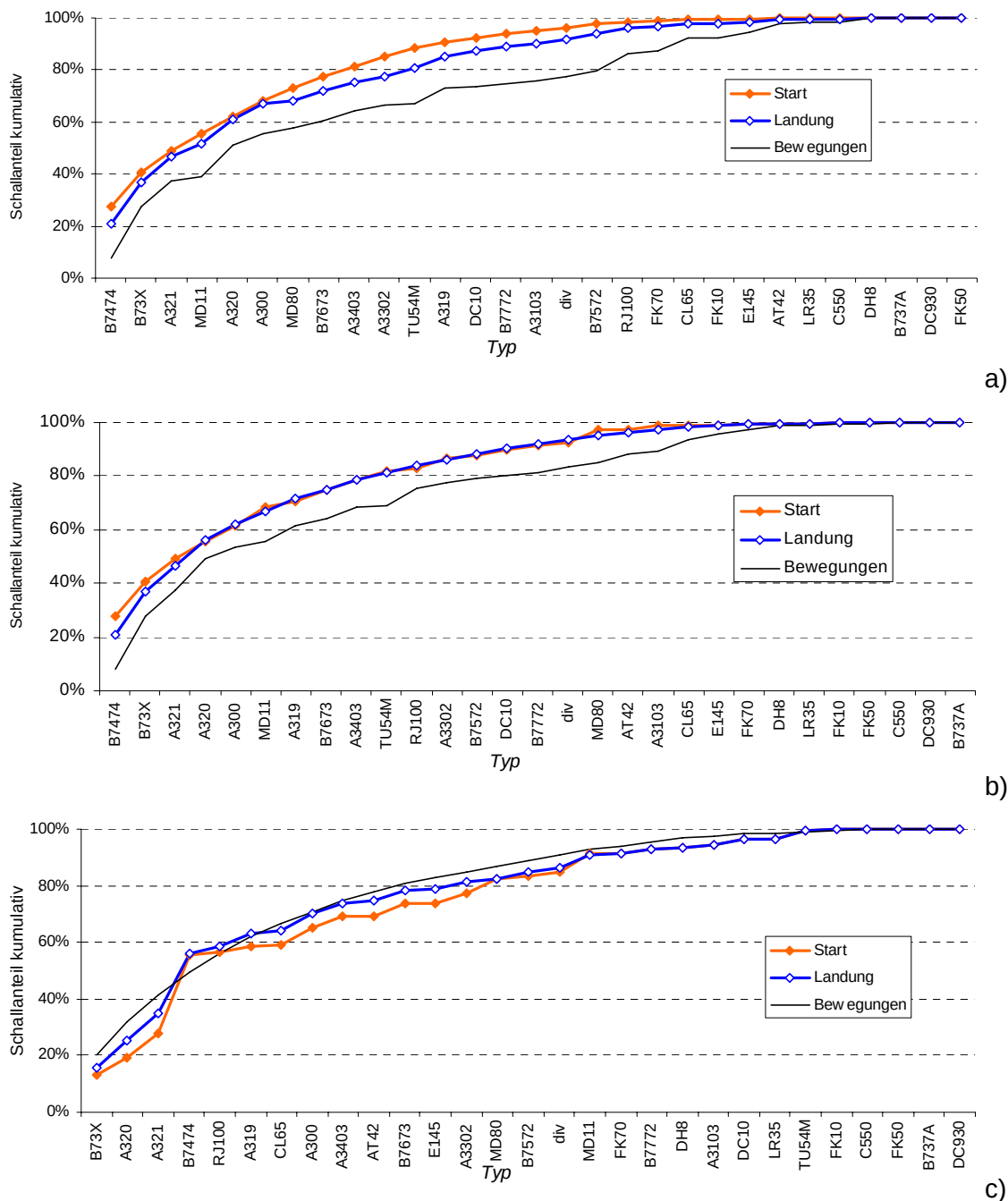
Abbildung 6 Kumulative Summe der Schallanteile pro Flugzeugtyp, sortiert nach Schallanteil Start (a), Landing (b) und Anzahl Bewegungen (c)
