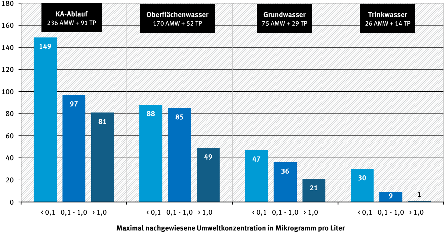
Anzahl detektierter Wirkstoffe und Transformationsprodukte inkl. Metabolite
