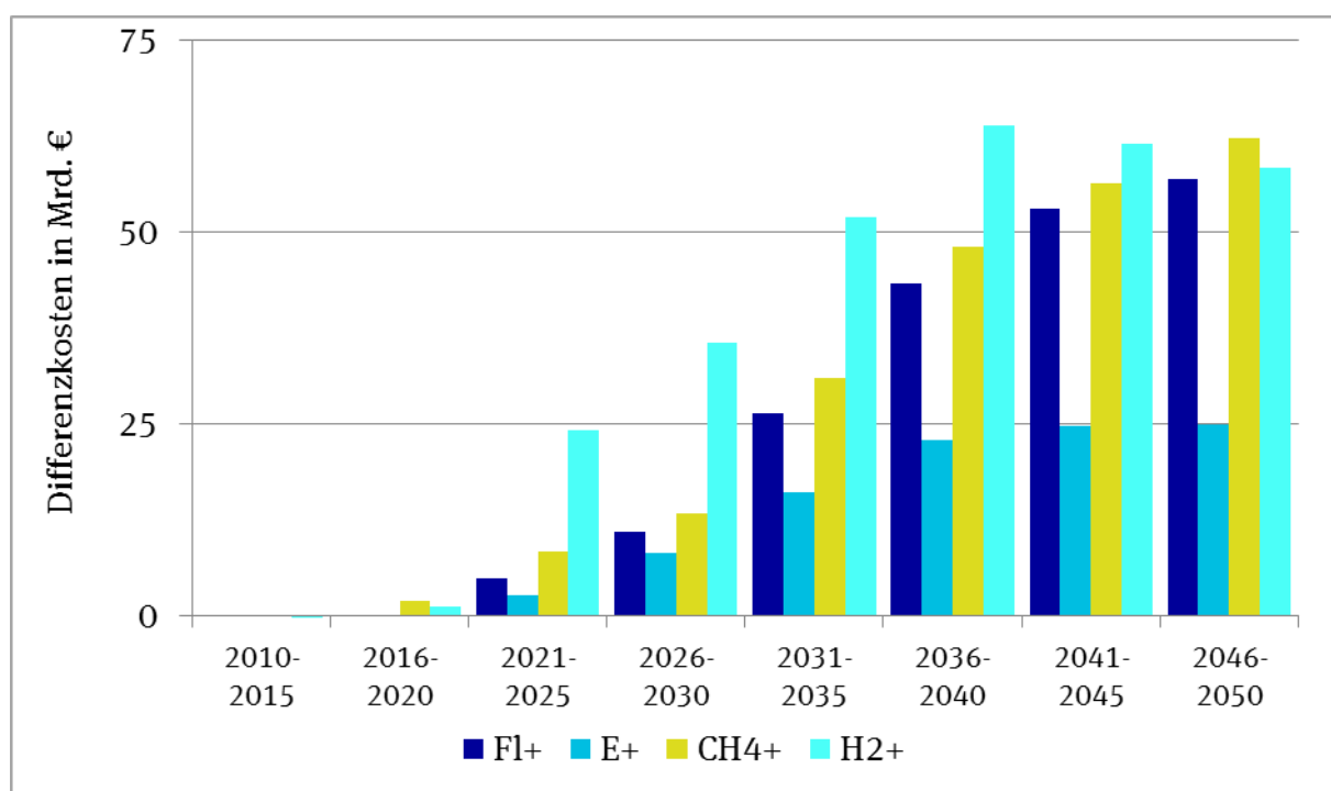
Abbildung 3-4: Straßenfernverkehr: Differenzkosten im Vergleich zum Referenz-Szenario in Fünffjahresschritten (positiv: Mehrkosten)
