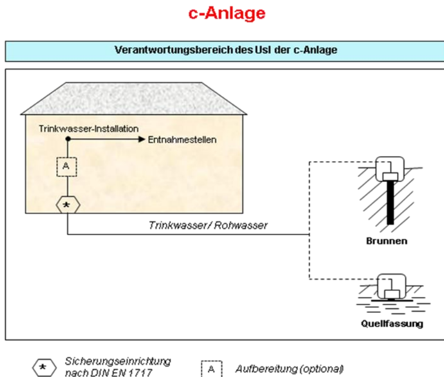
Abb. 1: Verantwortungsbereich des USI einer c-Anlage für die eigene Versorgung
