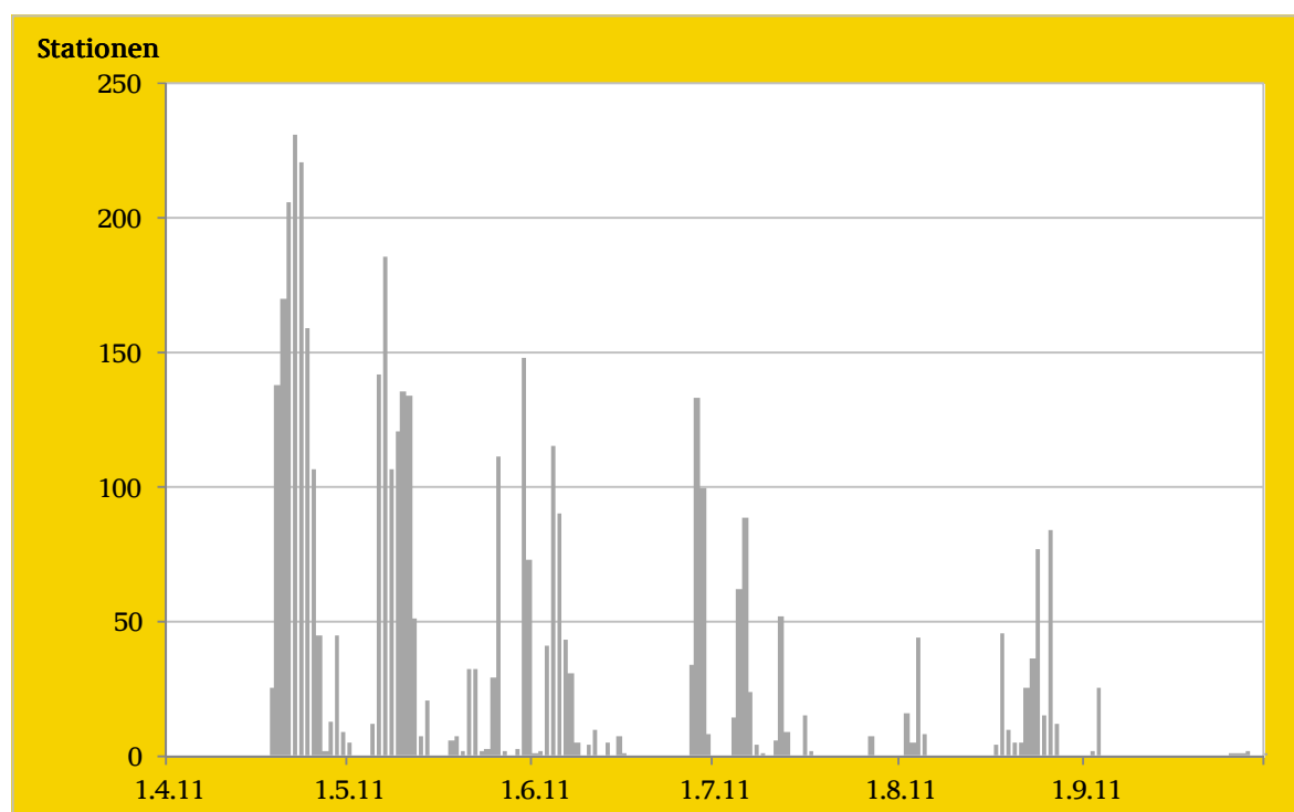
Abbildung 2: Zahl der Stationen mit einem höchsten täglichen 8-Stunden-Mittelwert über 120 \mu\text{g}/\text{m}^3 in den Monaten April bis September.
