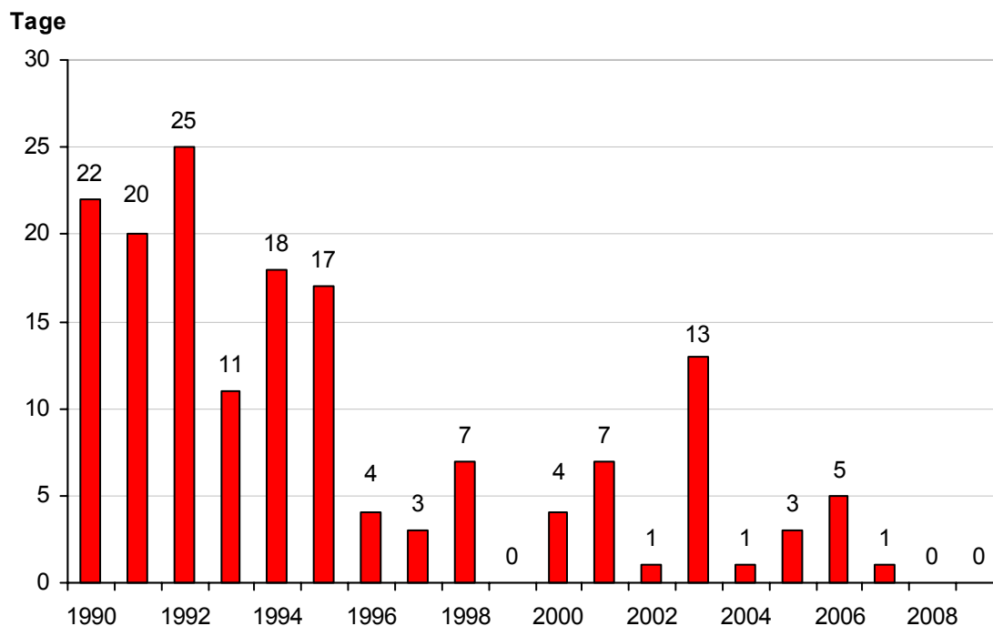
Abbildung 1: Zahl der Tage mit Ozonkonzentrationen über 240 µg/m 3 in den Jahren 1990 bis 2009
