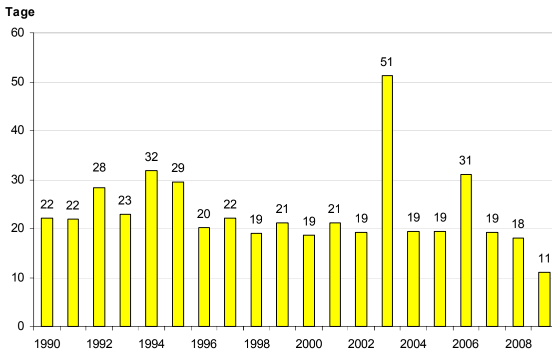
Abbildung 5: Zahl der Tage, an denen 8-h-Mittelwerte größer als 120 \mu\text{g}/\text{m}^3 auftraten; Mittel über die Zahl der Stationen des jeweiligen Jahres
