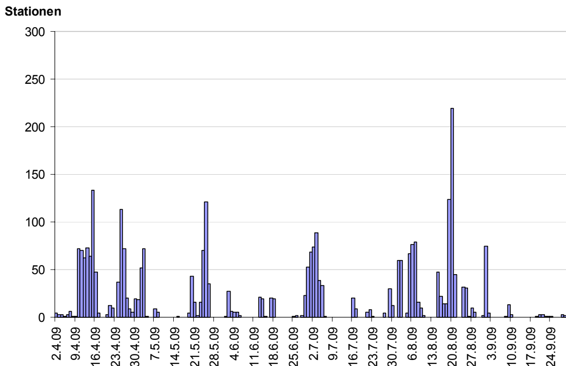
Abbildung 4: Zahl der Stationen mit einem höchsten täglichen 8-Stunden-Mittelwert größer als 120 µg/m³
