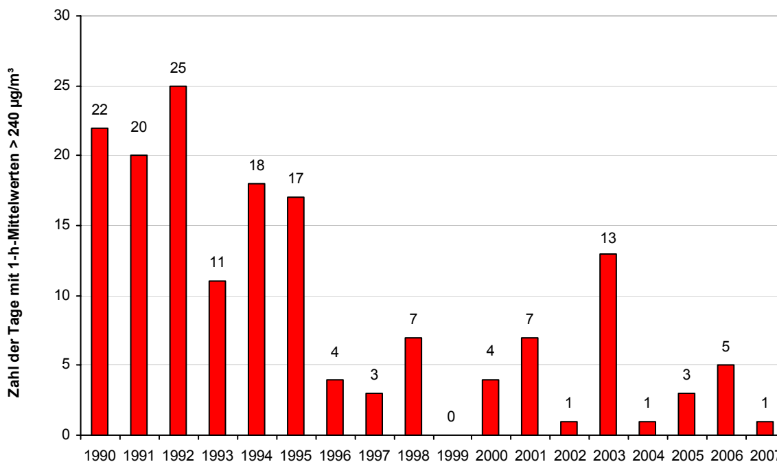
Abbildung 1: Zahl der Tage mit Ozonekonzentrationen über 240 µg/m³ in den Jahren 1990 bis 2007
