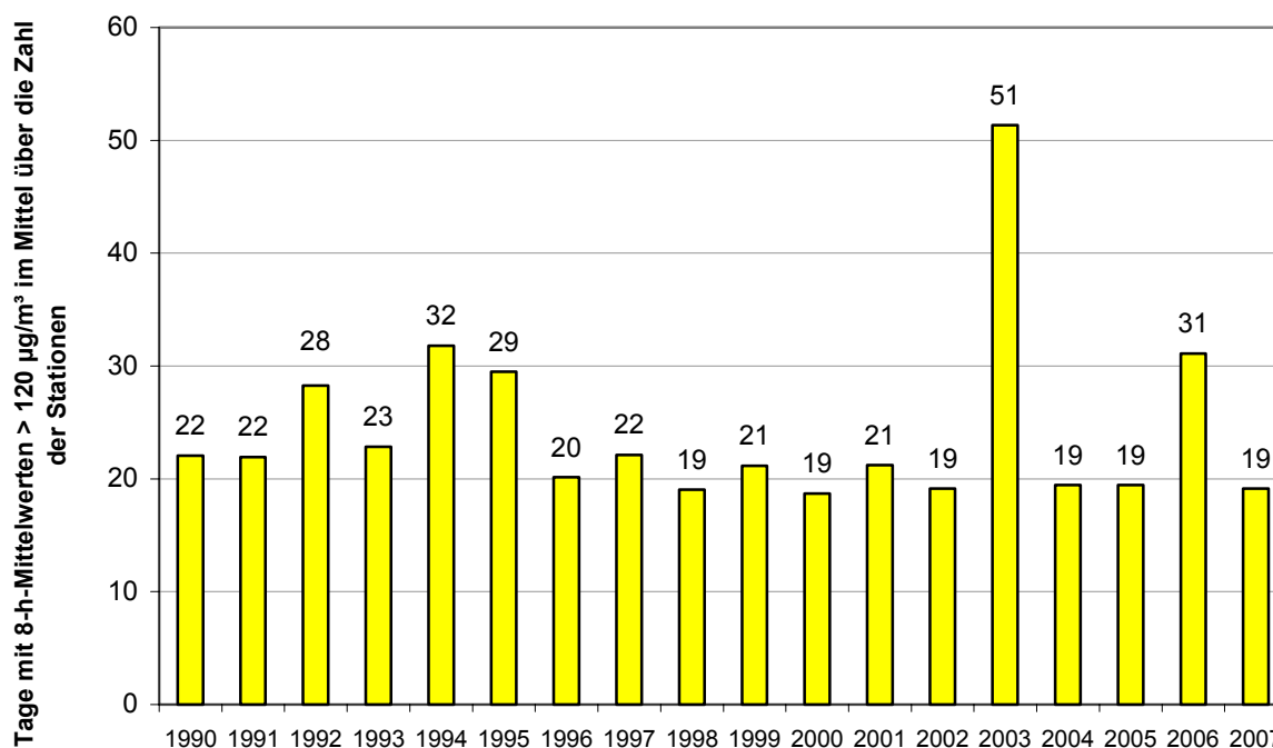
Abbildung 5: Zahl der Tage, an denen 8-h-Mittelwerte größer als 120 µg/m³ auftraten; Mittel über die Zahl der Stationen des jeweiligen Jahres
