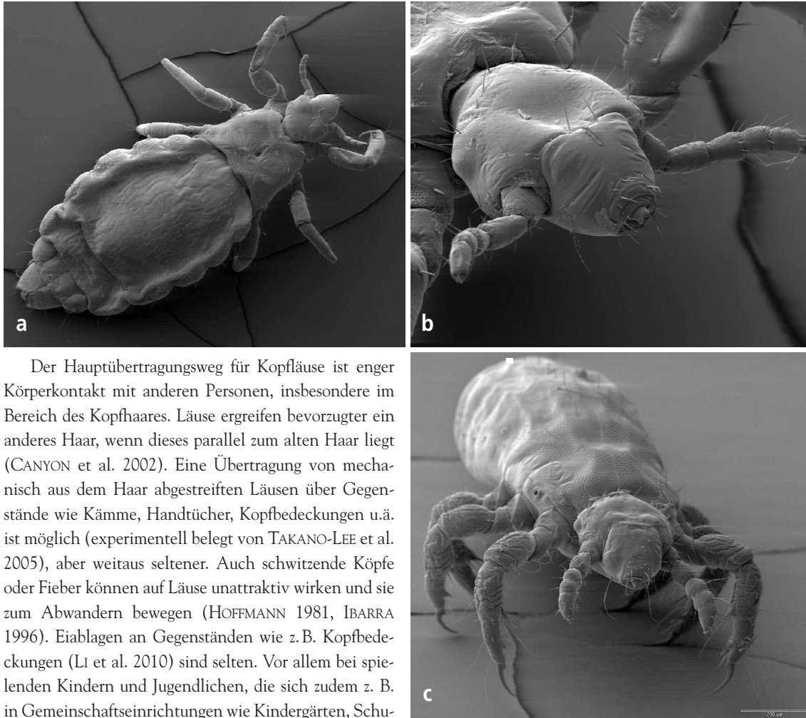
Abb. 3: Kleiderlaus-Stadien: (a) Weibchen und (b) Kopf des Weibchens, (c) erstes Juvenilstadium.
