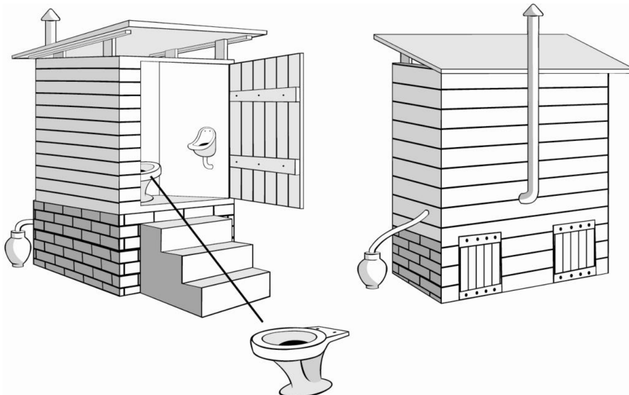
рис. 1. Внешний вид сухого туалета.
