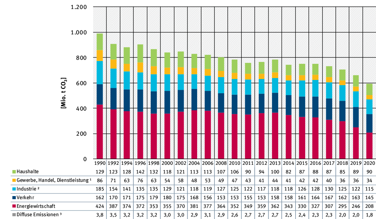
Abbildung 4: Entwicklung der energiebedingten CO 2 -Emissionen 1990-2020
