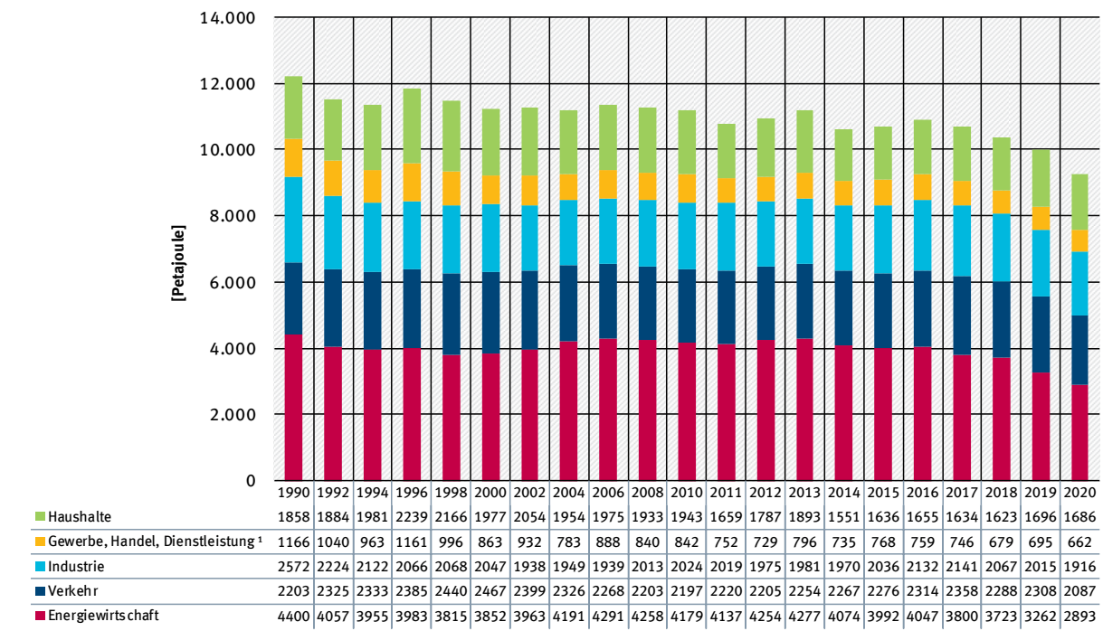
Abbildung 1: Entwicklung der Brennstoffeinsätze nach Quellgruppen 1990-2020
