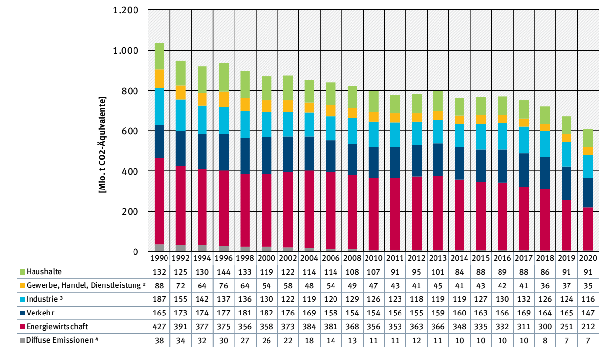
Abbildung 2: Entwicklung der energiebedingten THG-Emissionen 1 1990-2020
