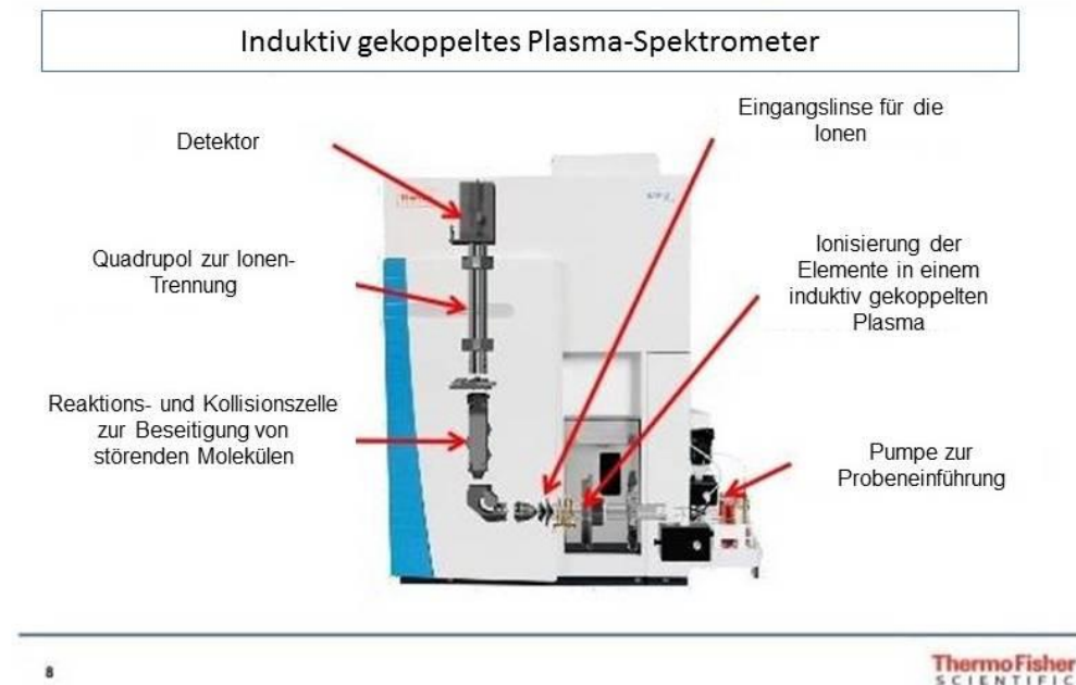
Abbildung 8: Ionenflussdiagramm des ICP-MS Geräts der Fa. Thermo Scientific, Modell iCAP RQ
