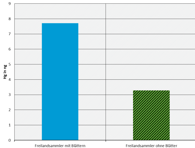
Abbildung 33: Hg-Auslaugung aus den in die Sammeltrichter gefallenen Blättern während der Streufallphase ermittelt unter Freilandbedingungen (AFS-Werte)
