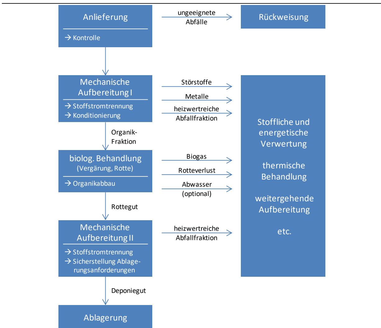
Abbildung 79: Stoffstromschema Mechanisch-Biologische Abfallbehandlung 207
