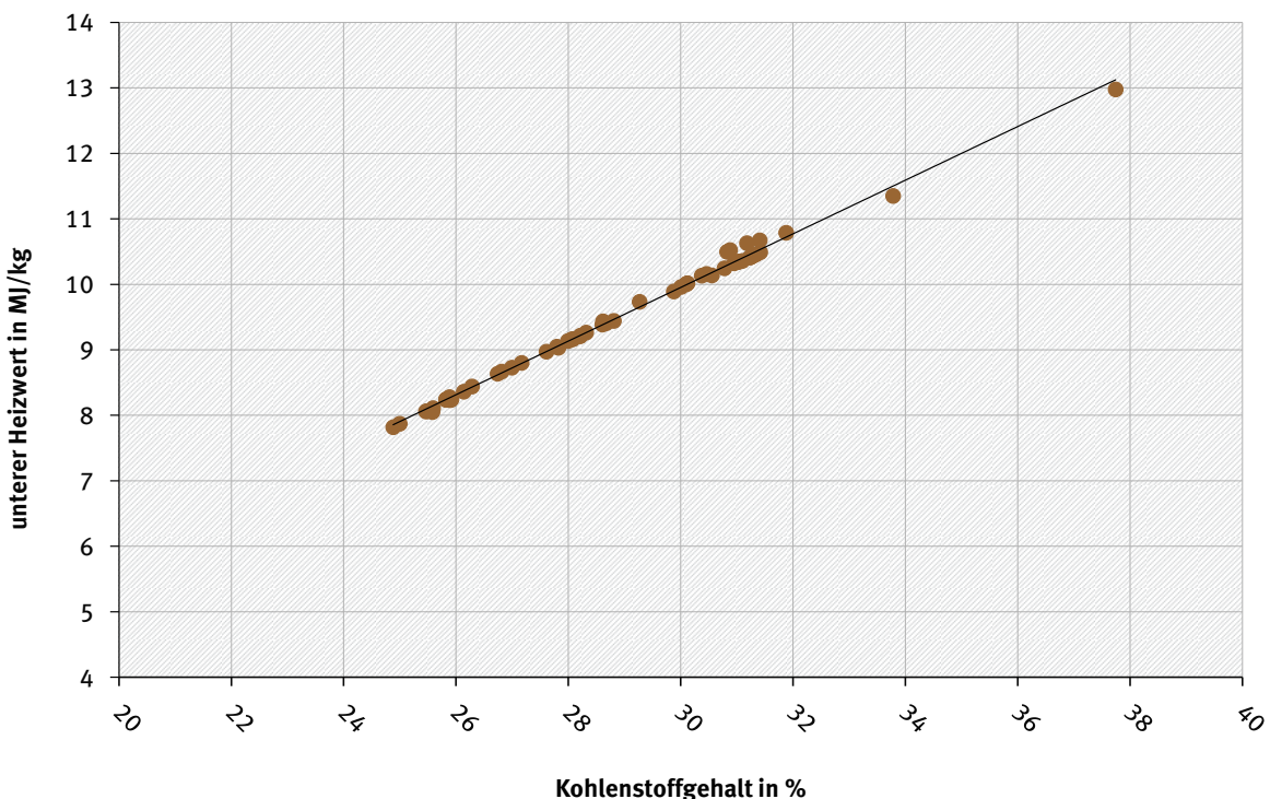
Abbildung 87: Verhältnis zwischen Kohlenstoffgehalten und Heizwerten am Beispiel einer Rohbraunkohlequalität
