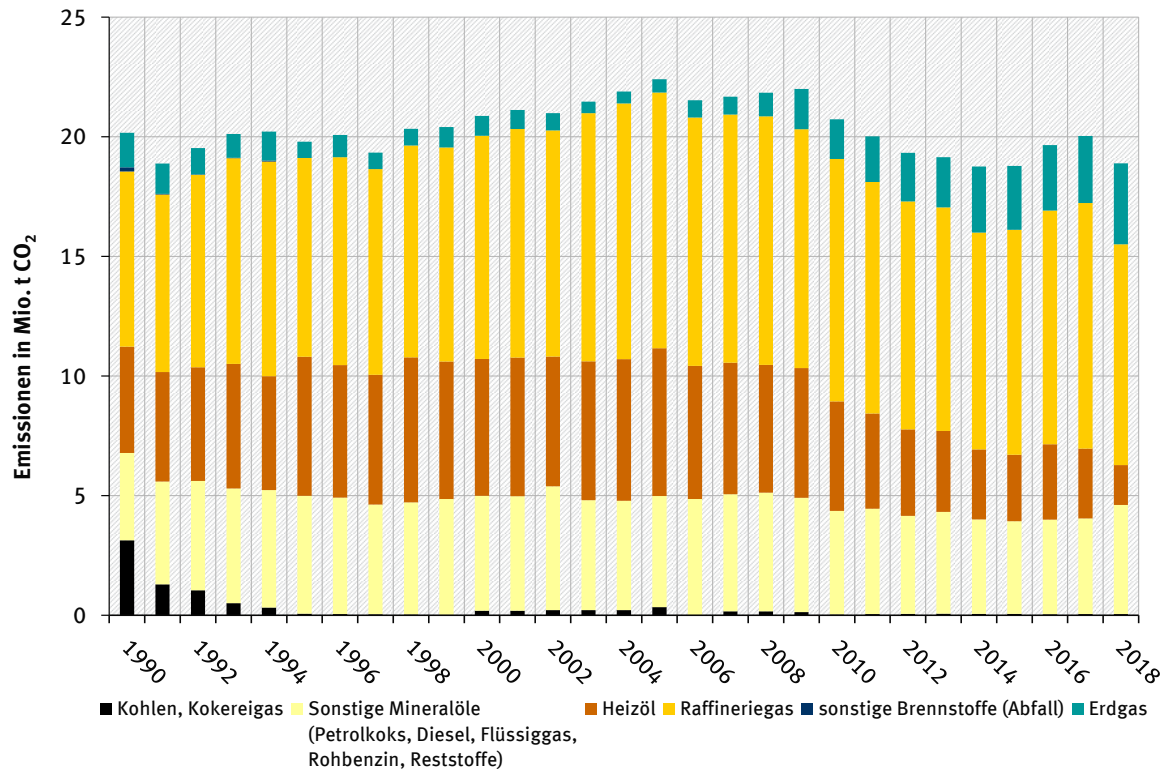
Abbildung 24: Entwicklung der CO 2 -Emissionen der Kategorie 1.A.1.b
