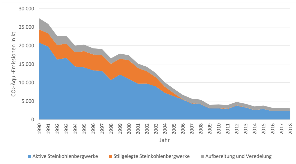
Abbildung 41: CO 2 -Äquivalentemissionen der Kategorie 1.B.1
