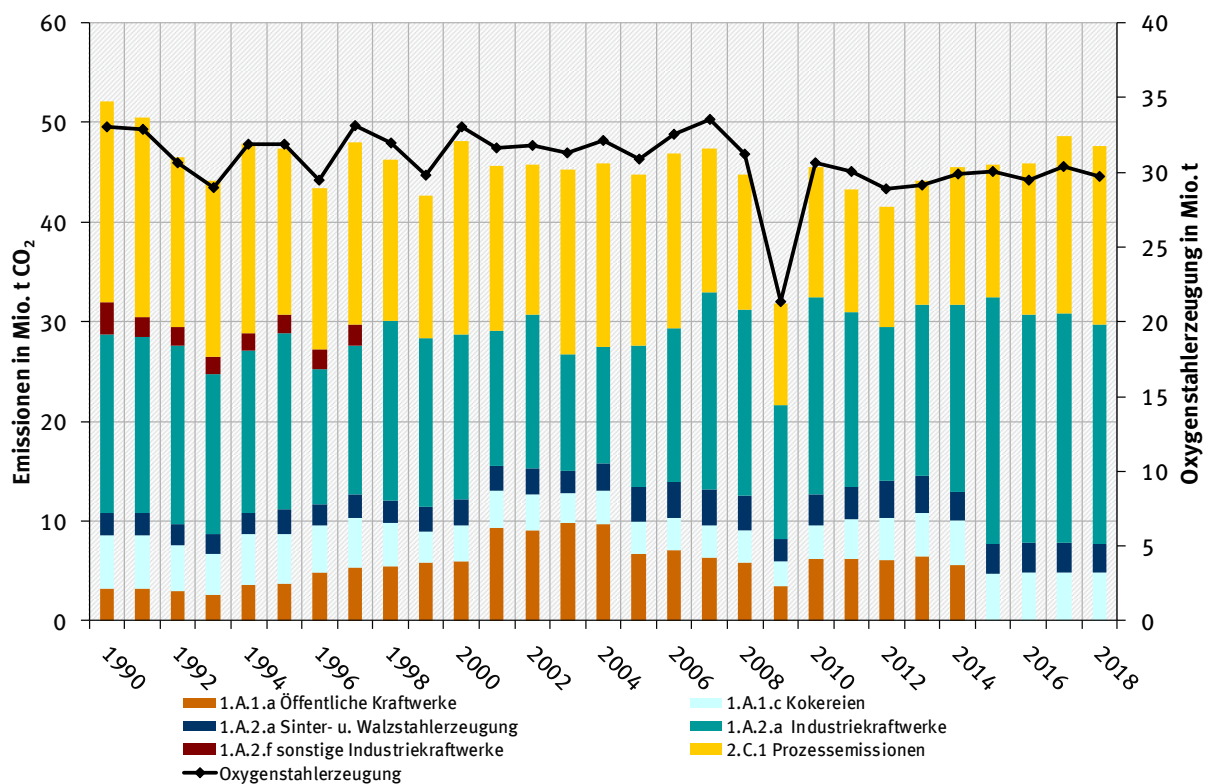
Abbildung 45: Zeitlicher Verlauf und Quellgruppenzuordnung der aus dem Reduktionsmitteleinsatz zur Primärstahlerzeugung bzw. Gichtgasaufkommen resultierenden CO 2 -Emissionen
