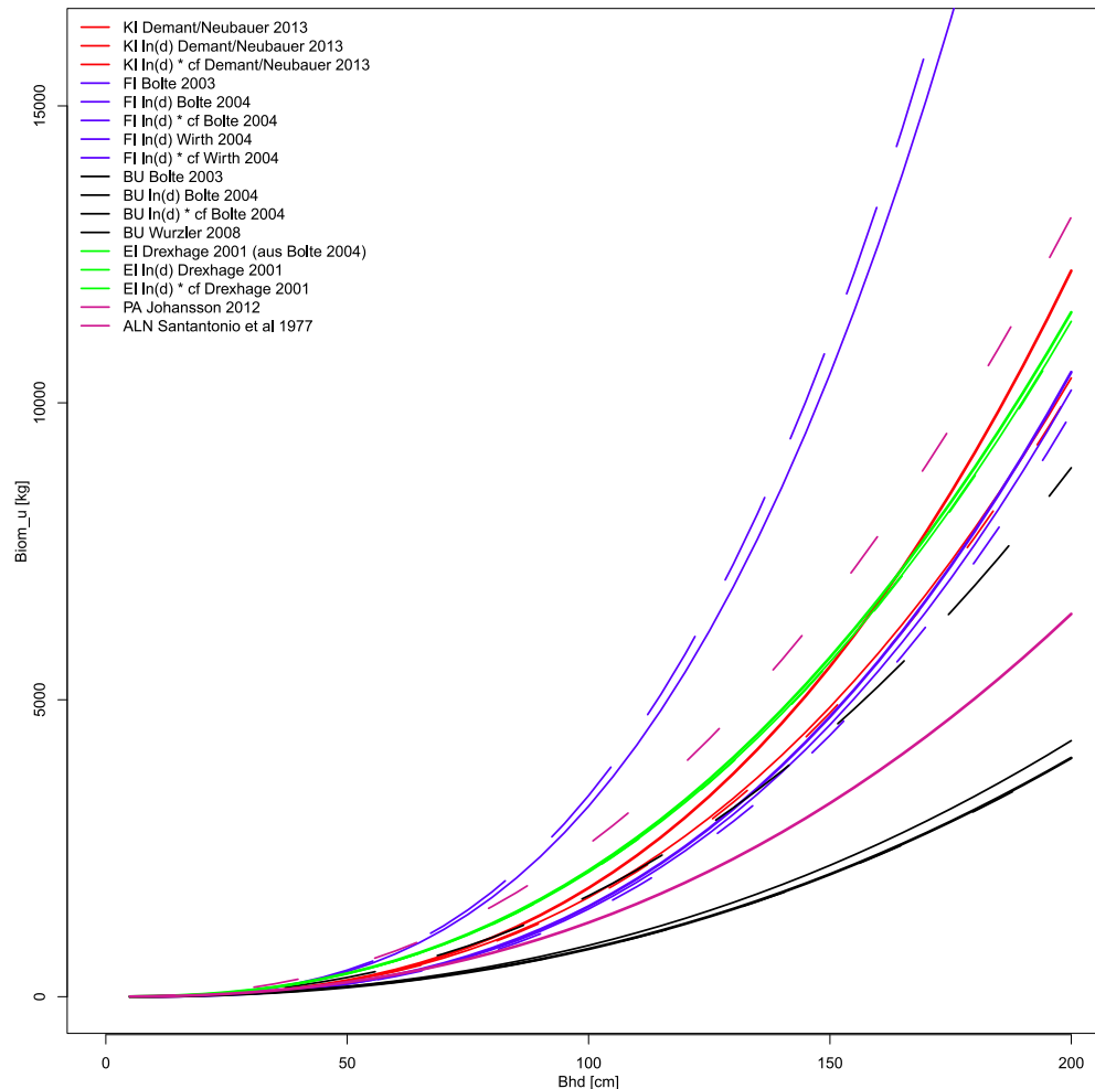
Abbildung 57: Vergleich verschiedener Funktionen zur Ableitung der unterirdischen Phytomasse
