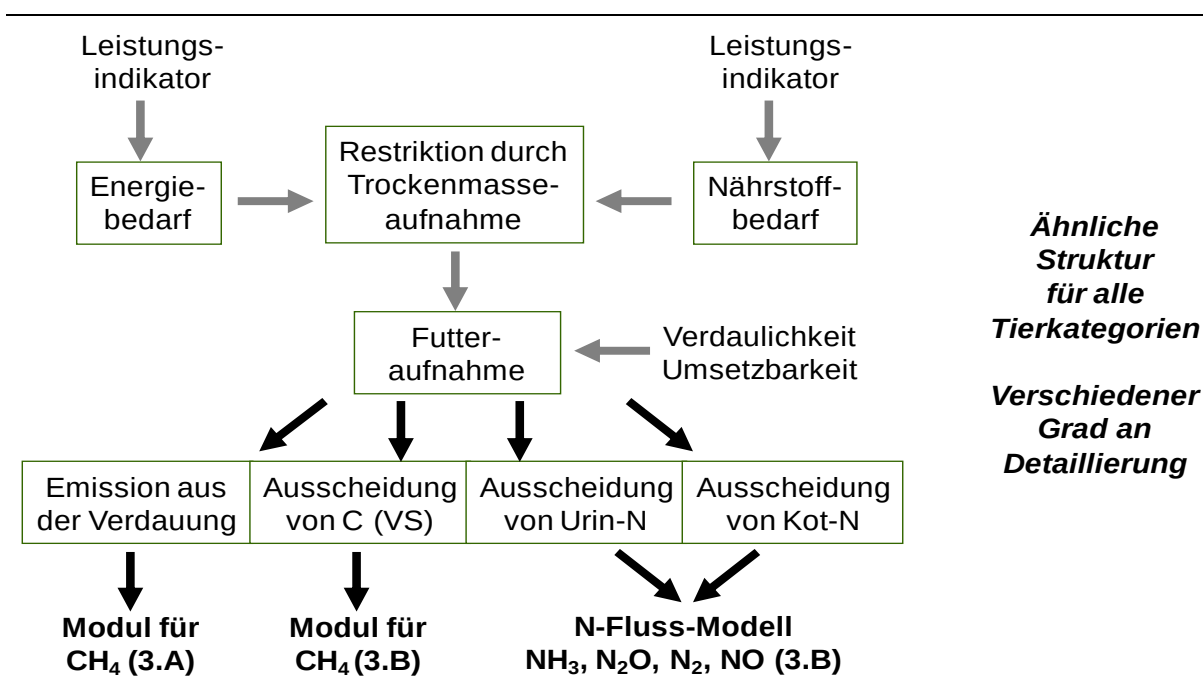
Abbildung 48: Logik der nationalen Methodik für die Emissionsberechnungen in der Tierhaltung am Beispiel der Milchkuh. („Leistungsindikator“ steht hier für die Summe aus leistungs- und erhaltungsbedingtem Bedarf.)
