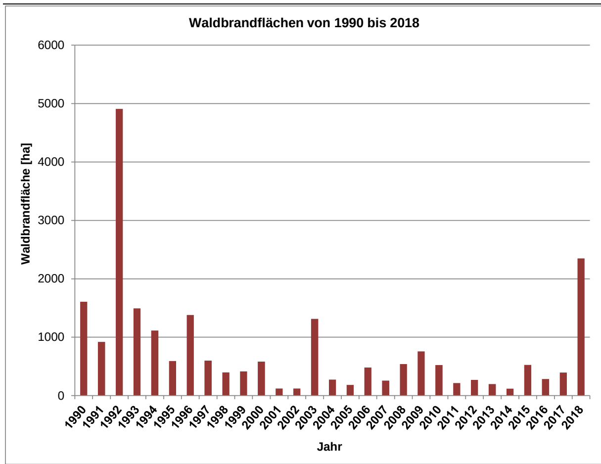
Abbildung 59: Waldbrandflächen zwischen 1990 und 2018 (nach BLE, 2019)
