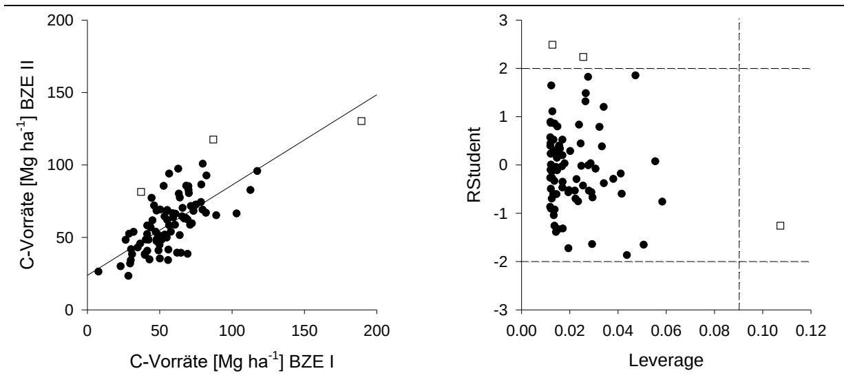
Abbildung 58: Regression zwischen Kohlenstoffvorräten (0-30cm) der BZE II und der BZE I (links) sowie die identifizierten Ausreißer anhand der Residuen-Analyse durch Student-Residuen und den "high leverage"-Punkten (rechts) am Beispiel einer Leitbodeneinheit
