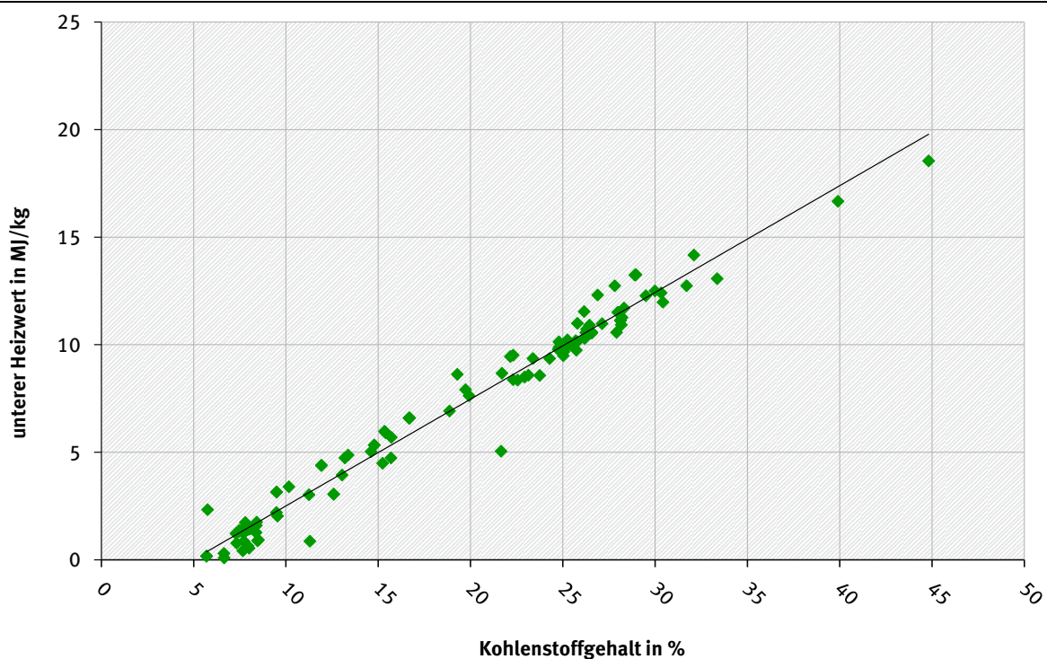
Abbildung 88: Verhältnis zwischen Kohlenstoffgehalten und Heizwerten für verschiedene Klärschlämme
