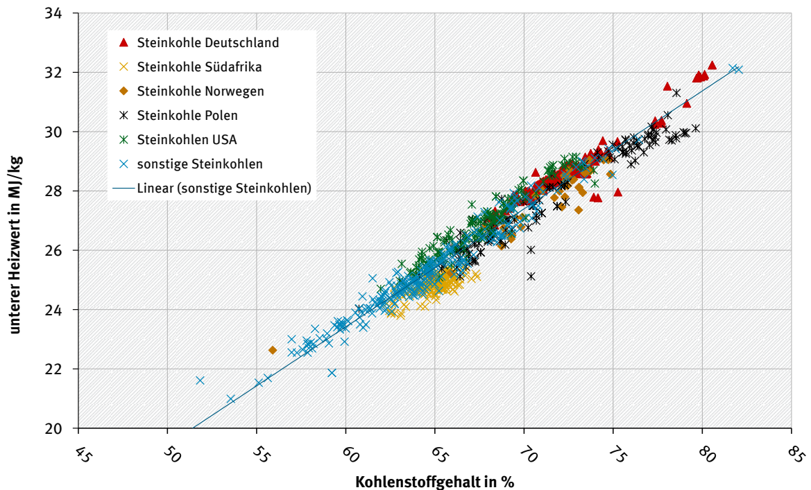
Abbildung 86: Verhältnis zwischen Kohlenstoffgehalten und Heizwerten für verschiedene Steinkohlenqualitäten
