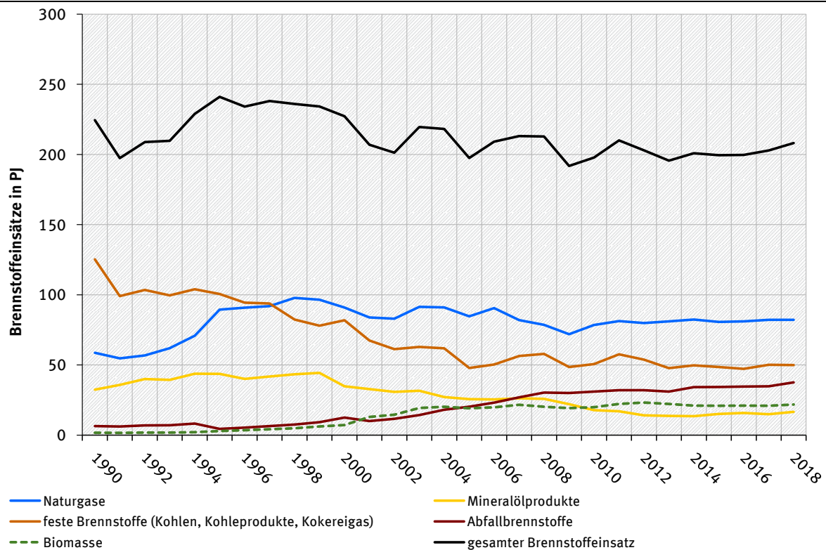
Abbildung 27: Entwicklung der Brennstoffeinsätze der Kategorie 1.A.2.f Non-Metallic Minerals
