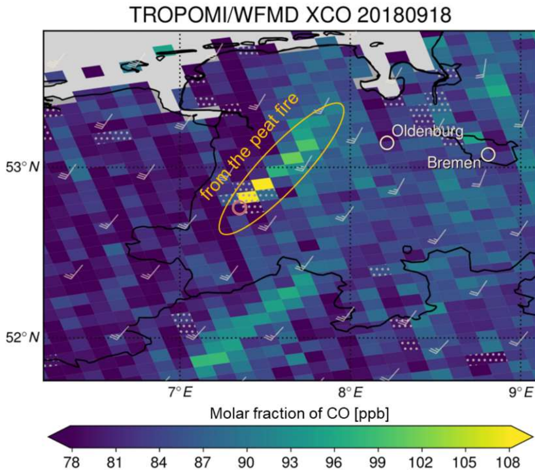
Abbildung 71: CO-Fahne des Moorbrands am 18.09.2018 (ESA Sentinel-5P) aus Schneising et al. (2019)
