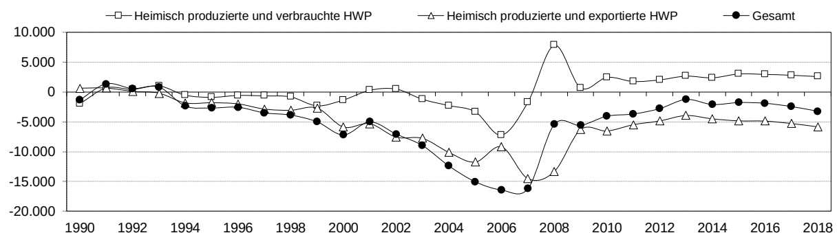
Abbildung 72: Netto CO 2 -Emissionen und Einbindungen in Holzprodukten [kt CO 2 ]
