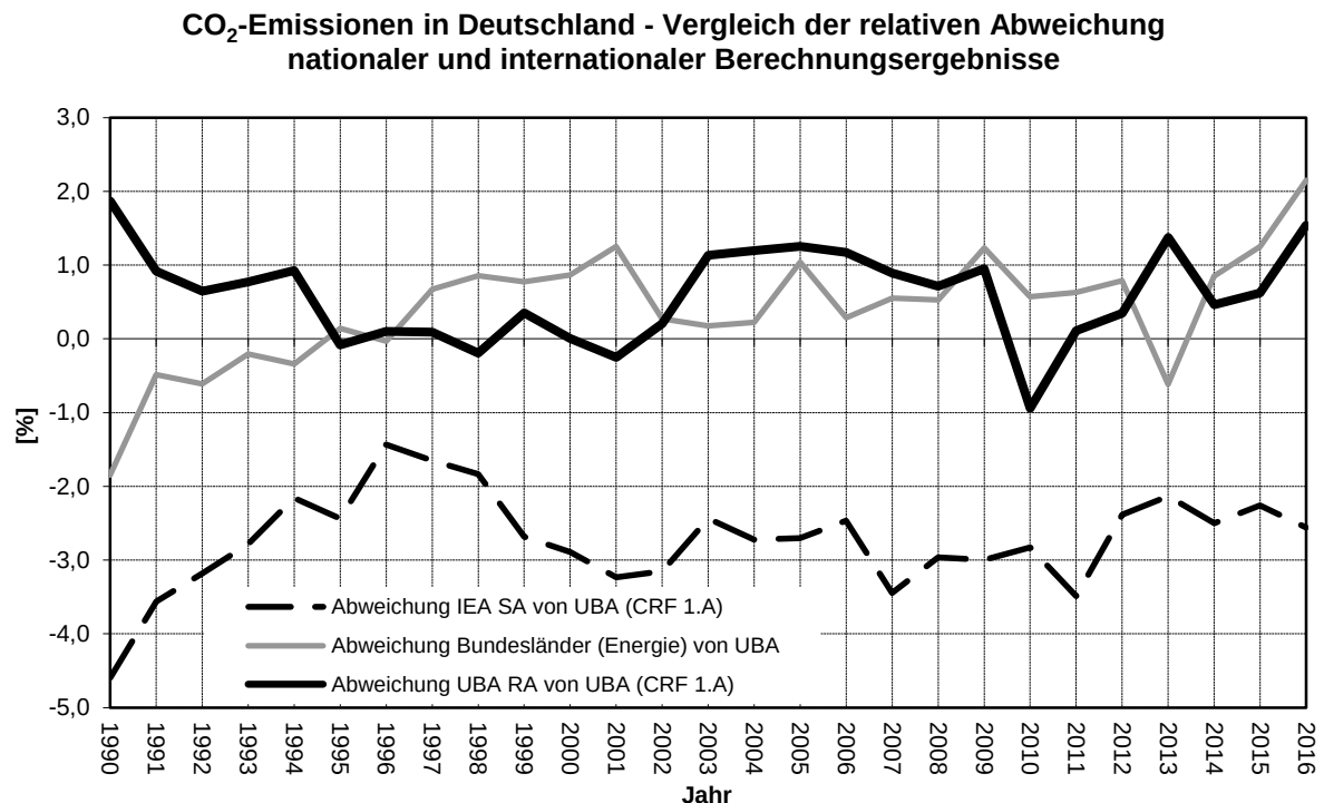
Abbildung 20: CO 2 -Emissionen in Deutschland – Vergleich der relativen Abweichungen nationaler und internationaler Berechnungsergebnisse (Stand NIR 2019)
