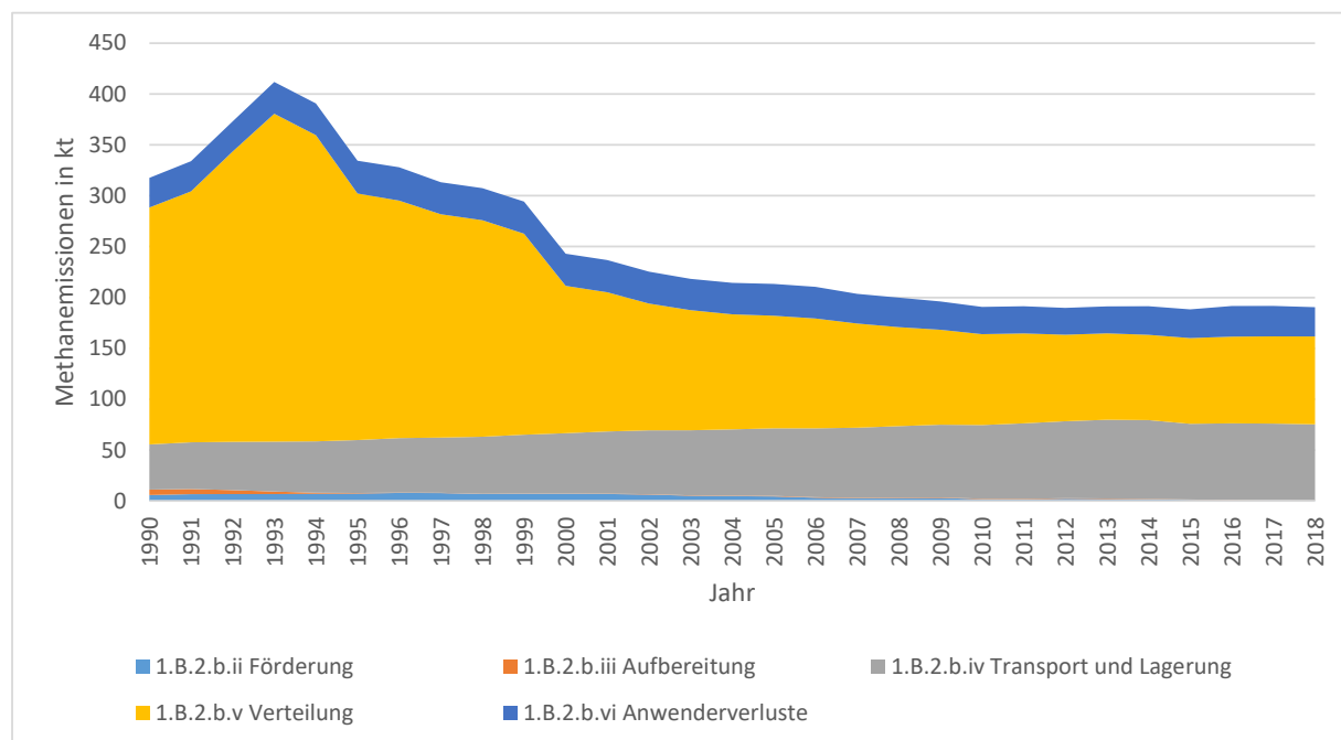
Abbildung 43: Entwicklung der Methanemissionen in 1.B.2.b seit 1990
