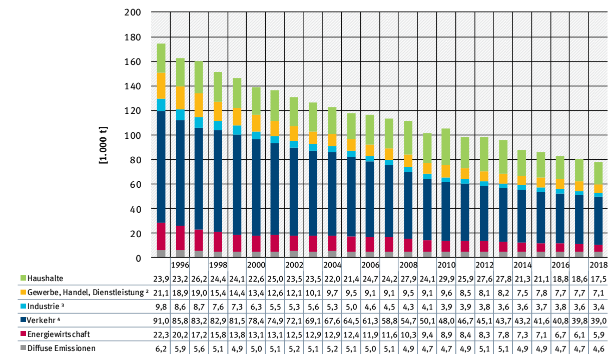
Abbildung 10: Entwicklung der energiebedingten Feinstaub-Emissionen 1 1995-2018
