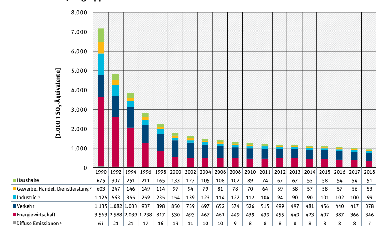
Abbildung 6: Entwicklung der energiebedingten Emissionen von Säurebildnern 1 nach Quellgruppen 1990-2018
