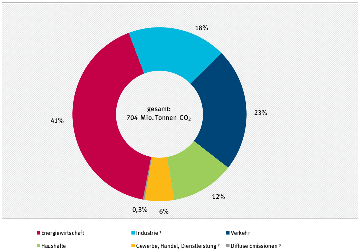
Abbildung 5: Anteile der Quellgruppen an den energiebedingten CO 2 -Emissionen im Jahr 2018
