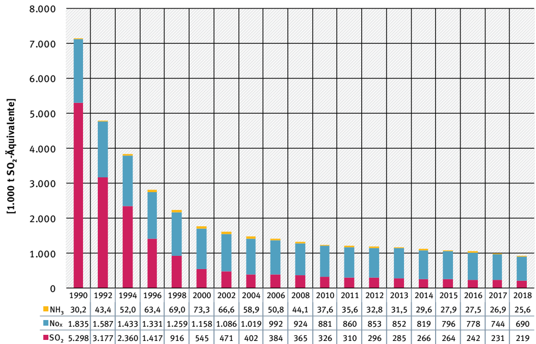
Abbildung 8: Entwicklung der energiebedingten Emissionen von säurebildenden 1 Luftschadstoffen 1990-2018
