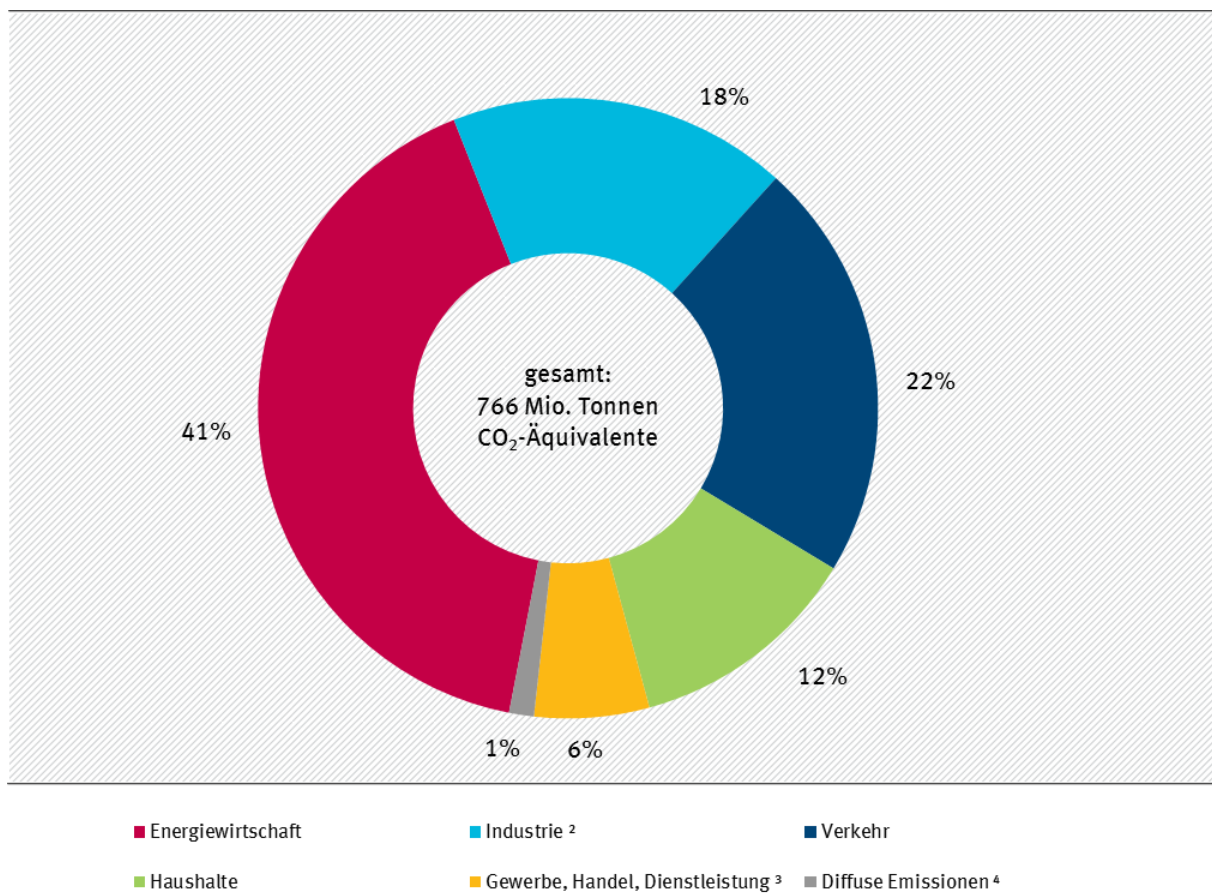
Abbildung 3: Anteile der Quellgruppen an den energiebedingten THG-Emissionen 1 im Jahr 2018
