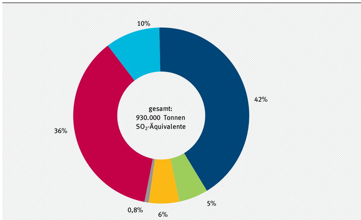
Abbildung 7: Anteile der Quellgruppen an den energiebedingten Emissionen von Säurebildnern 1 im Jahr 2018
