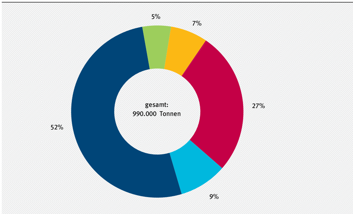
Abbildung 9: Anteile der Quellgruppen an den energiebedingten NO x -Emissionen im Jahr 2018
