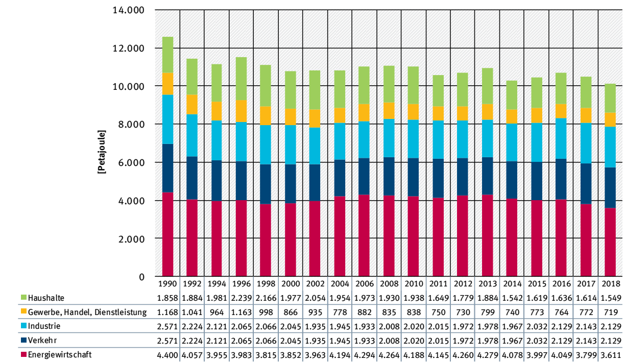
Abbildung 1: Entwicklung der Brennstoffeinsätze nach Quellgruppen 1990-2018
