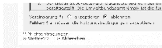
Fig. 5: Error message
