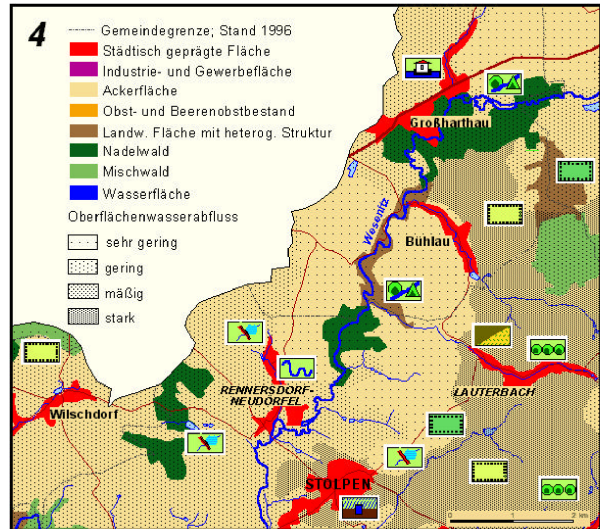
Abbildung 5: Flächennutzung, Oberflächenabfluss und Maßnahmenvorschläge zum Hochwasserschutz im Einzugsgebiet der Wesenitz
