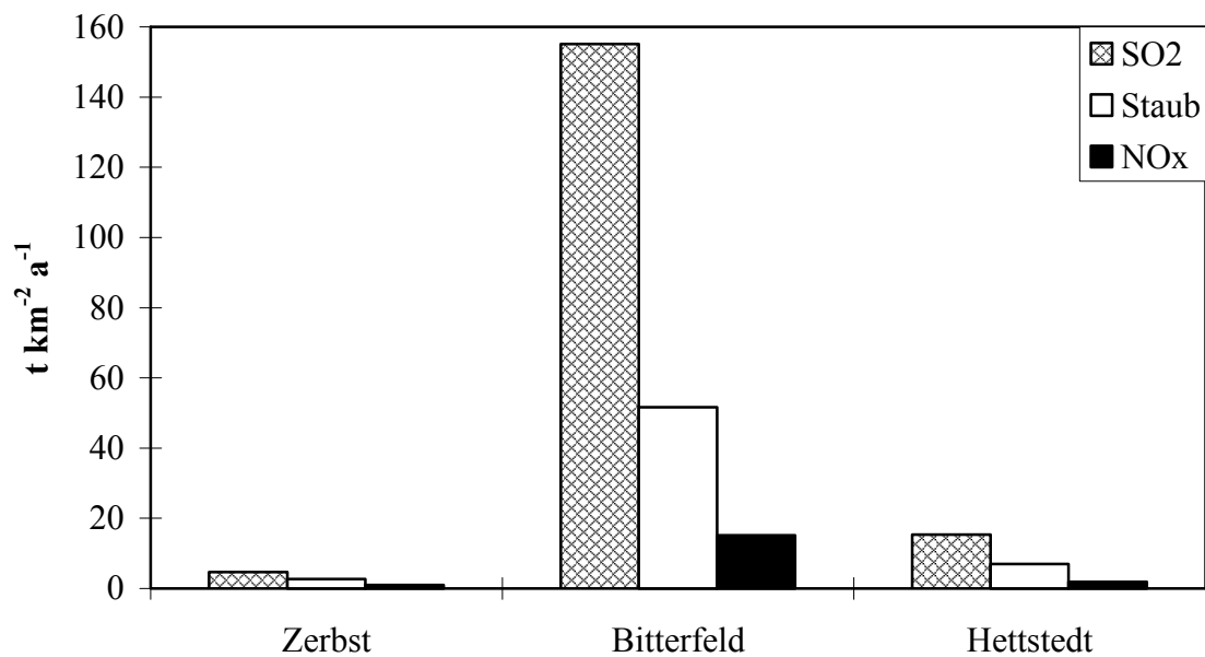
Abb. 2.4 Emissionen 1990 in t km -2 a -1 (Ministerium für Umwelt und Naturschutz des Landes Sachsen-Anhalt, 1990)
