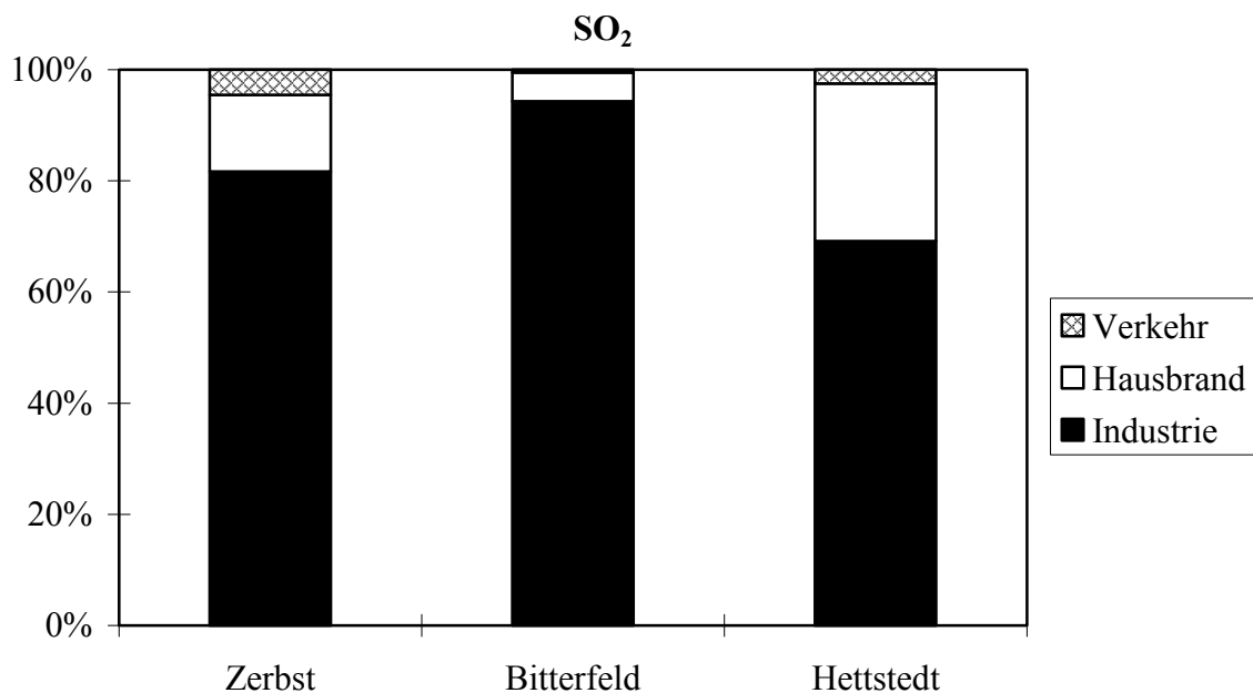
Abb. 2.5 Anteile der einzelnen Emittentengruppen an der Gesamtemission von SO 2 im Jahr 1990 für die Landkreise Anhalt-Zerbst, Bitterfeld und Hettstedt (Ministerium für Umwelt und Naturschutz des Landes Sachsen-Anhalt, 1990)
