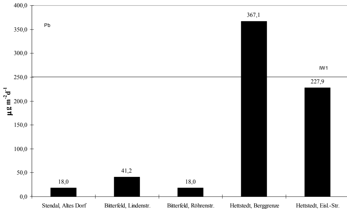
Abb. 2.2 Pb-Gehalt im Staubniederschlag - Jahresmittelwerte 1992 (in µg m -2 d -1 ) (Landesamt für Umweltschutz Sachsen-Anhalt, 1993). Die Daten von Stendal dienen als Anhaltswerte für Anhalt-Zerbst
