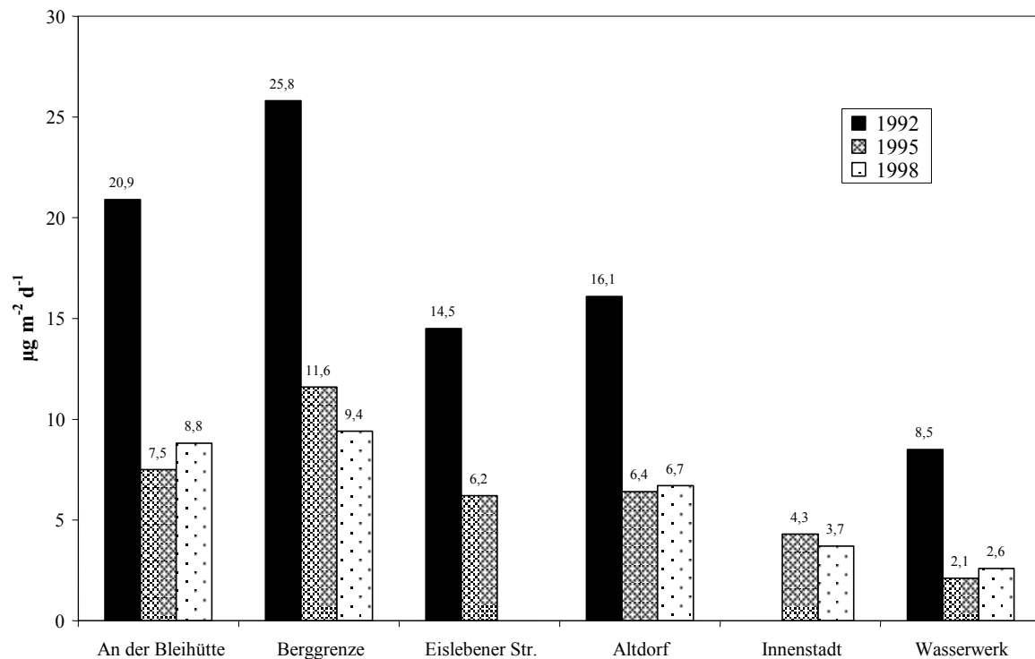
Abb. 2.10 Nickelgehalt im Staubniederschlag an unterschiedlichen Messstationen in Hettstedt - Jahresmittelwerte 1992, 1995, 1998 (in \mu\text{g m}^{-2} \text{d}^{-1} ) (Landesamt für Umweltschutz, 1993, 1996, 1999)
