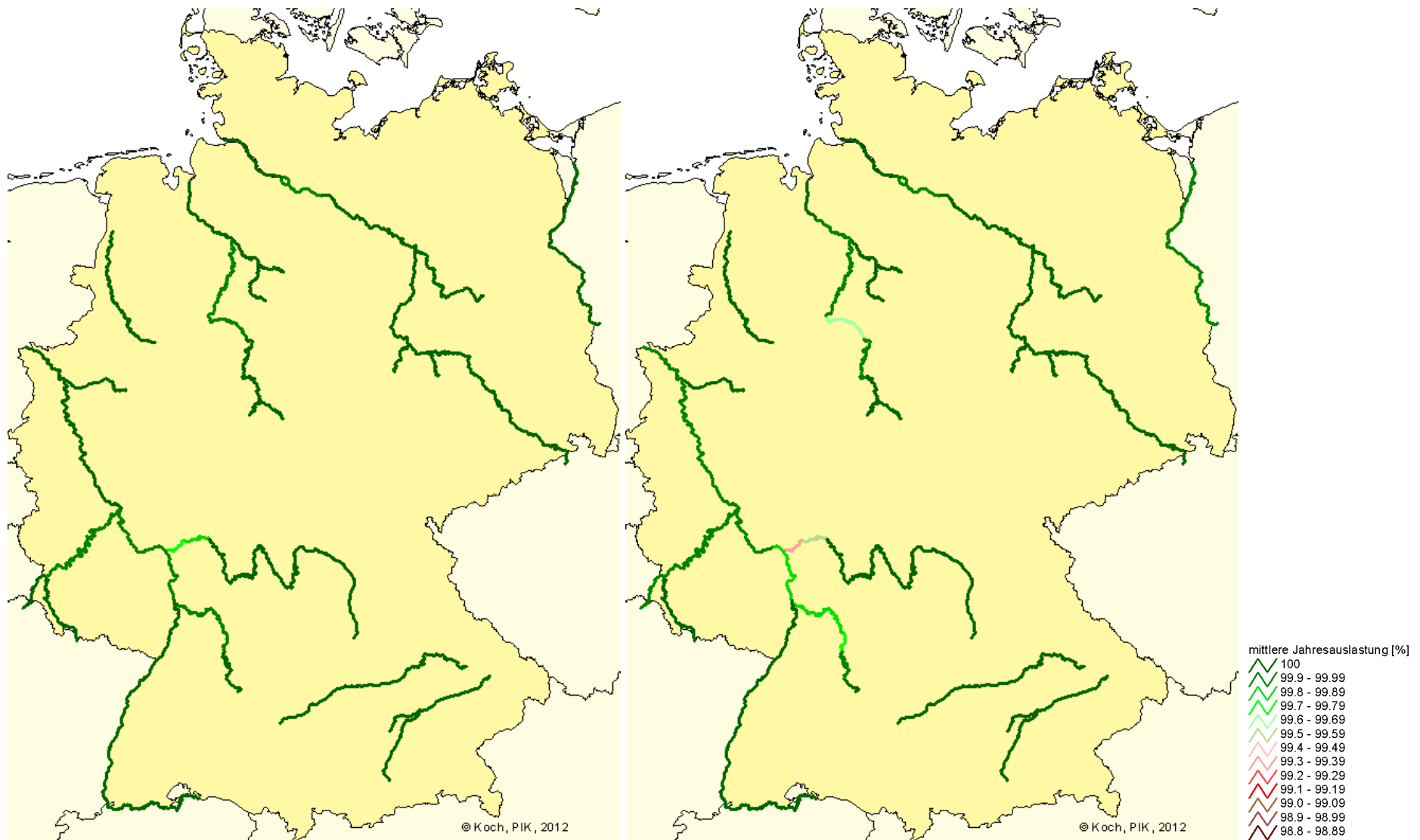
Abbildung 17: Mittlere Jahresauslastung thermischer Kraftwerke mit Kreislaufkühlung für 2010 (links) und unter dem 1K-Szenario für 2055 (rechts).
