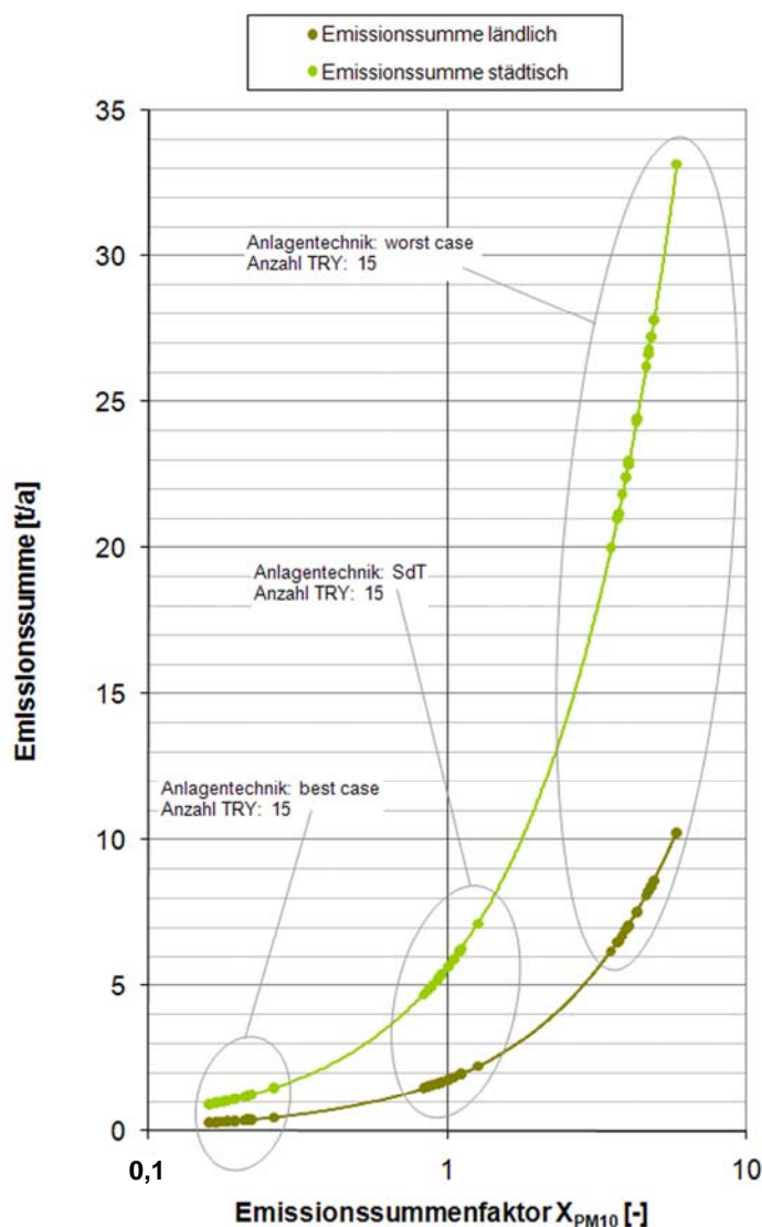
Bild 6-1 Zusammenhang zwischen Jahresemissionssummen für PM10 und Emissionssummenfaktoren für die beiden Modellgebiete am Beispiel Pelletkessel
