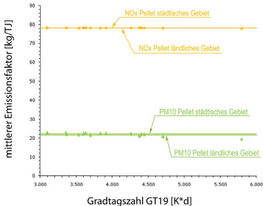
Bild 3-79 Jahresmittelwerte der Emissionsfaktoren \text{NO}_x und \text{PM}_{10} für Pelletfeuerungen in Abhängigkeit von der Gradtagszahl
