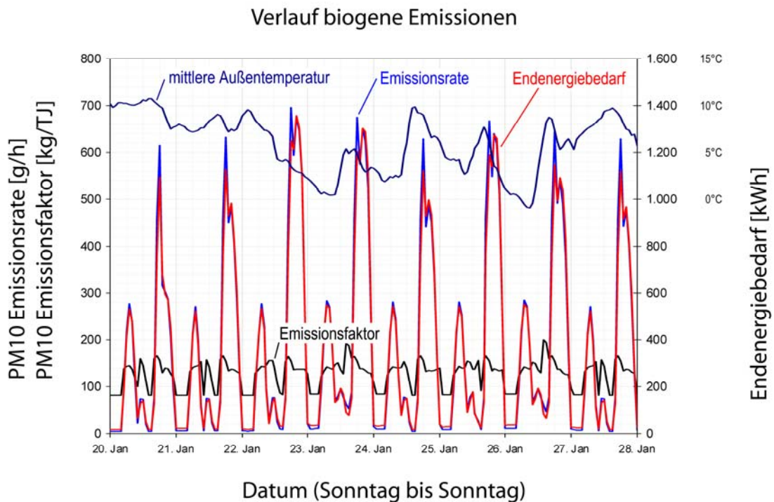
Bild 5-10 Verlauf der Emission aus Holzfeuerungen im Validierungsgebiet für den Zeitraum vom 20. bis 28. Januar 2008
