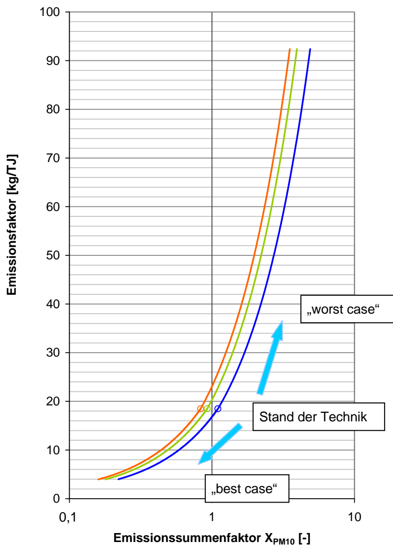
Bild 6-3 Zusammenhang zwischen Eingangsemissionsfaktor bei stationärem Betrieb bei Nennwärmeleistung für PM10 und Emissionssummenfaktor am Beispiel der Pelletfeuerungen für die Temperaturregion 3 (grün), 8 (blau) und 12 (rot)
