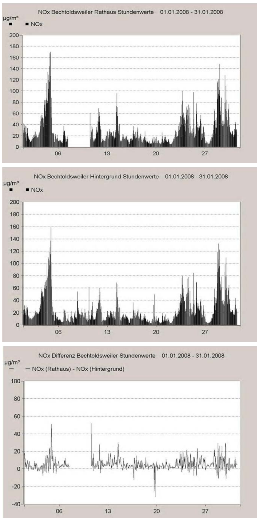
Bild 5-21 Verläufe der \text{NO}_x -Konzentrationen am Rathaus, im Hintergrund und die Differenz (Rathaus minus Hintergrund), Januar 2008
