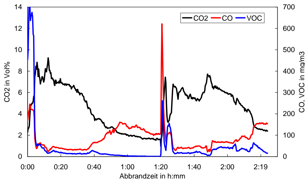
Bild 3-16 Typische Verläufe der CO 2 -, CO- und VOC-Konzentrationen beim Abbrand von Buchenscheitholz in einem Kaminofen
