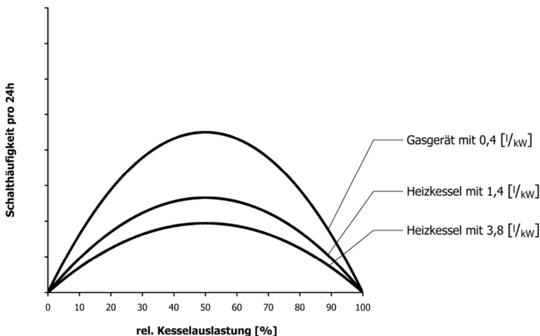
Bild 3-9 Qualitativer Zusammenhang der Start/Stopp-Vorgänge bezogen auf 24 h in Abhängigkeit von der relativen Kesselauslastung und des Kesselwasserinhalts (Struschka et al., 2000)
