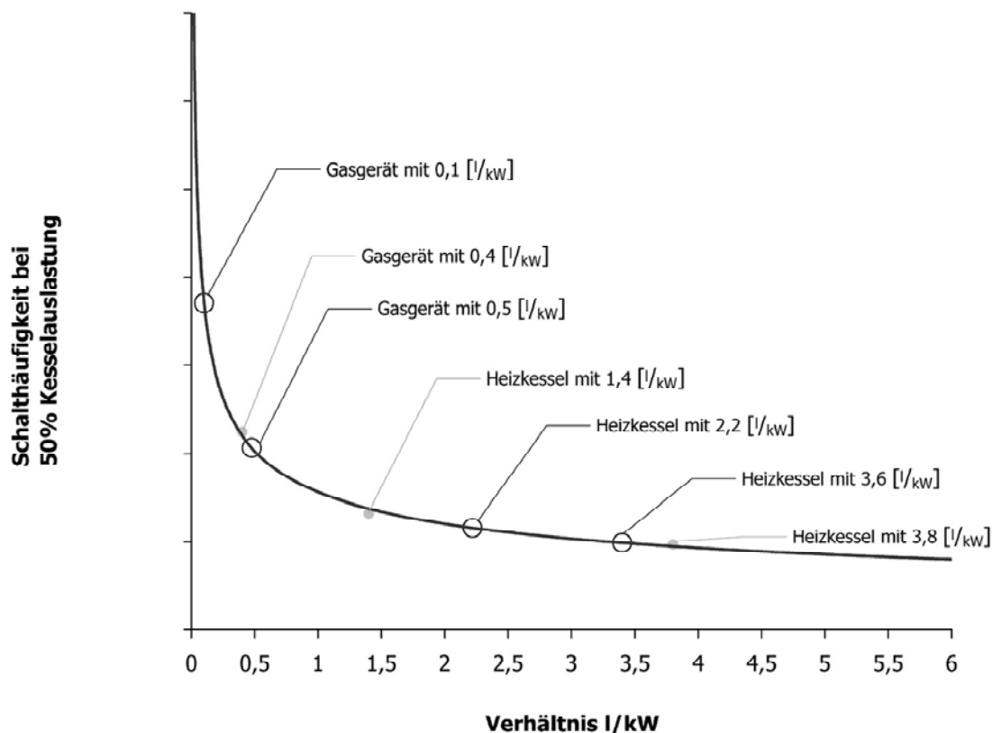
Bild 3-10 Qualitativer Zusammenhang der Schalthäufigkeit bei 50 % relativer Kesselauslastung für unterschiedliche Kesselwasserinhalte zu Nennwärmeleistungsverhältnisse ( l/kW -Verhältnisse)
