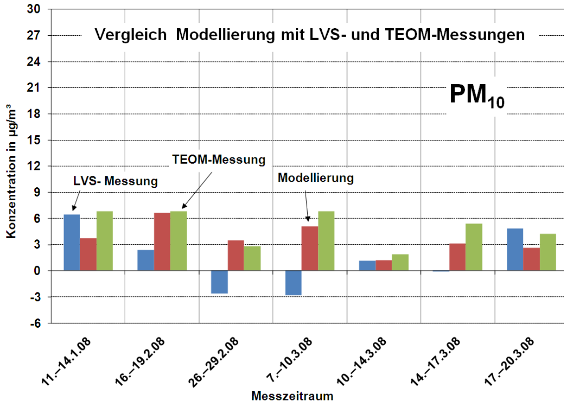
Bild 5-36 Vergleich modellierter, gravimetrisch (mit Low Volume Sammlern – LVS) und mit den TEOM-Geräten bestimmter mittlerer PM10-Zusatzbelastungen. Die Mittelungszeit ist durch gravimetrisch bedingte Sammelzeiten bestimmt: 3 – 4 Tage, Filterwechsel jeweils Nachmittags
