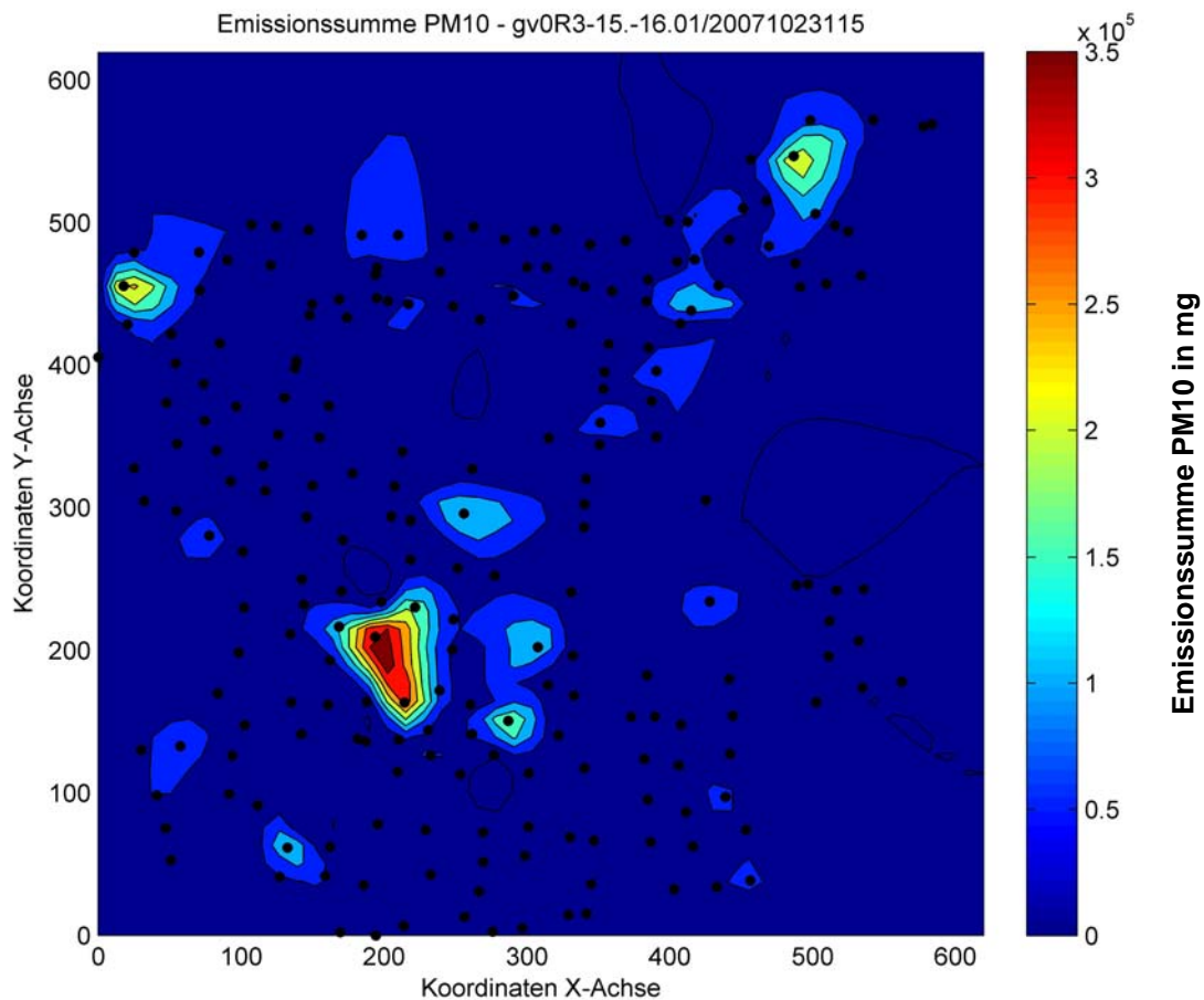
Bild 5-13 Berechnete PM10-Emissionsverteilung für eine Situation in Bechtoldswiler (räumlich interpoliert)
