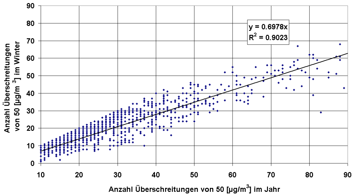
Bild 6-16 Anzahl der Tage mit mehr als 50 µg/m 3 im Winter im Vergleich zu Anzahl der Tage im Jahresmittel für die Jahre 2001 bis 2005
