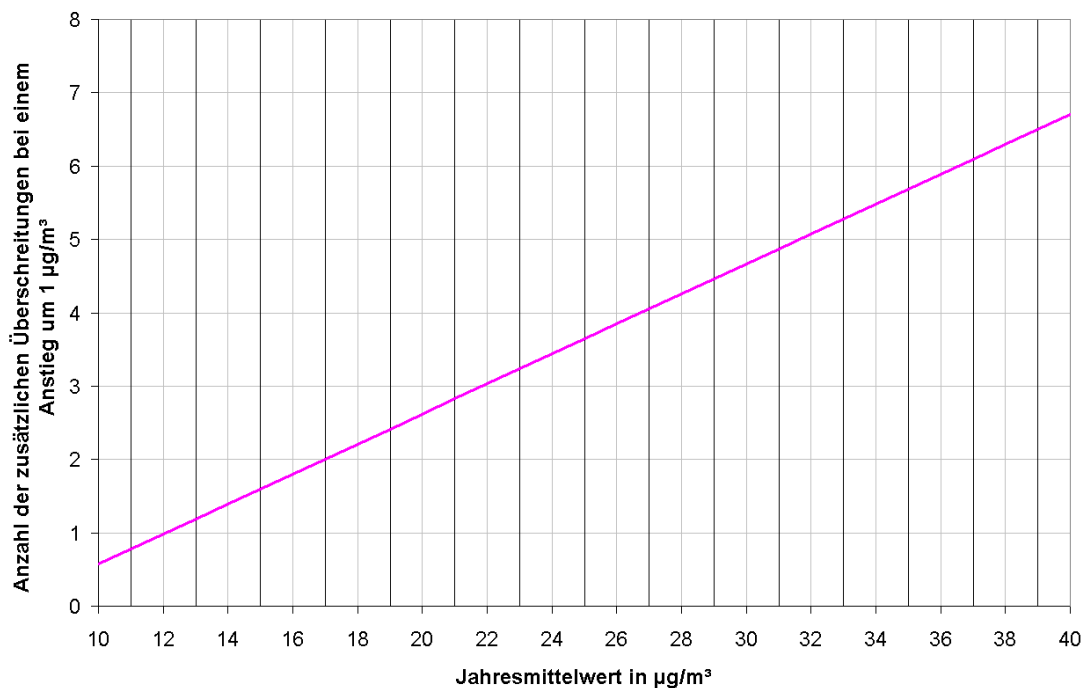
Bild 6-17 Zunahme der Anzahl der Überschreitungen bei Anstieg des Jahresmittelwerts um 1 µg/m 3 in Abhängigkeit von der absoluten Höhe des Jahresmittelwerts
