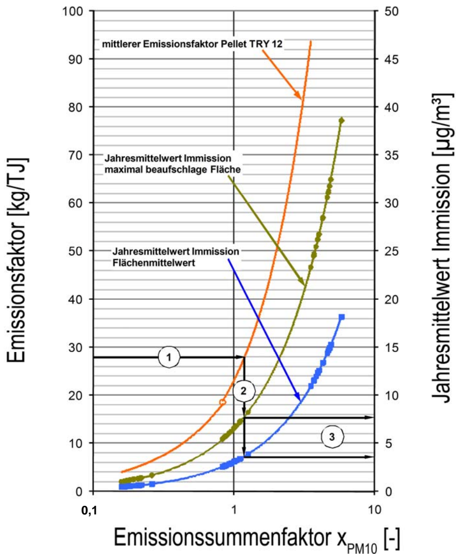
Bild 6-4 Zusammenhang zwischen Emissionssummenfaktor und Eingangsemissionsfaktor sowie Immissionsjahresmittelwert für PM 10 am Beispiel der Pelletfeuerungen für die Temperaturregion TRY 12 (weitere Randbedingungen: ländliches Modellgebiet, Quellhöhe auf First und AKTerm Stuttgart, Endenergiebedarf zu 100 % mit Pellets gedeckt)
