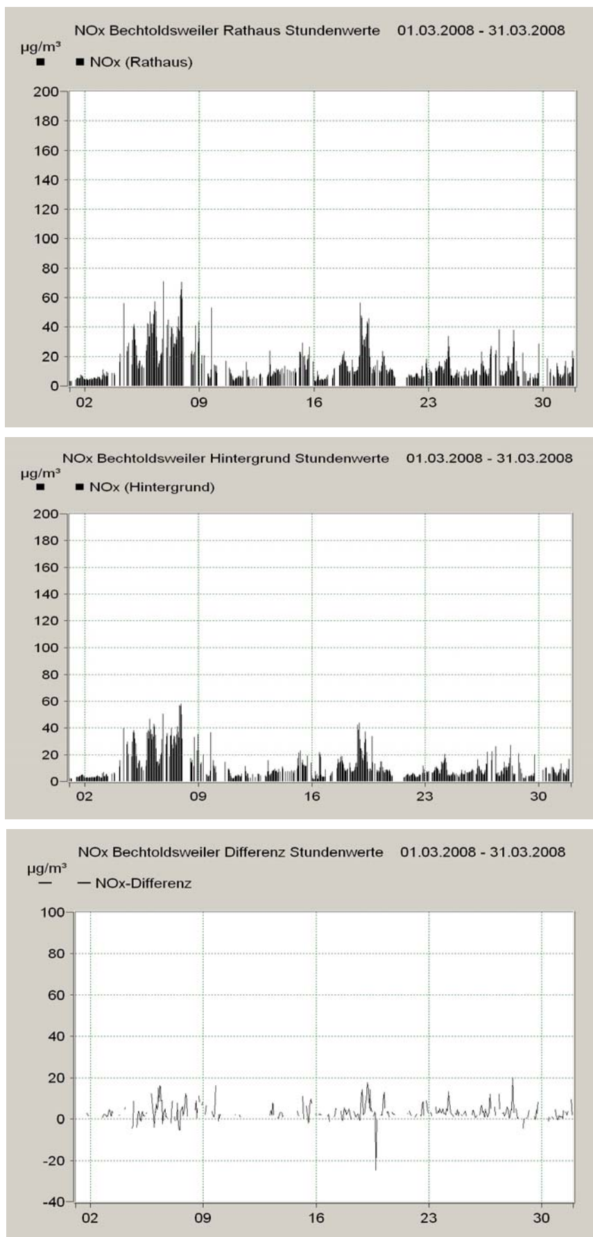
Bild 5-27 Verläufe der NO x -Konzentrationen am Rathaus, im Hintergrund und die Differenz (Rathaus minus Hintergrund), März 2008
