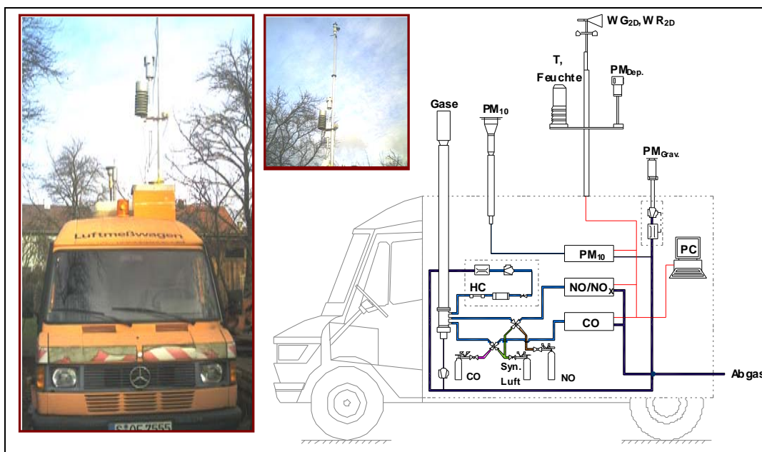
Bild 5-18 Anordnung der Messtechnik an der Station Rathaus (Messwagen)
