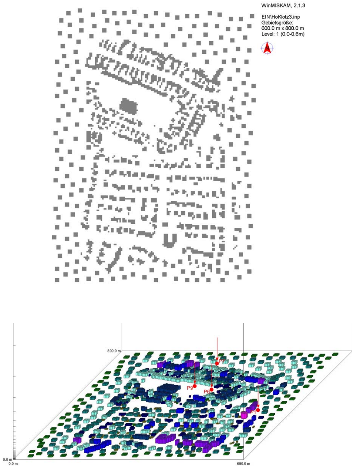
Bild 4-7 Ländliches Untersuchungsgebiet mit Umgebungsrauigkeiten und Auswertepunkten (Fall HoK13)
