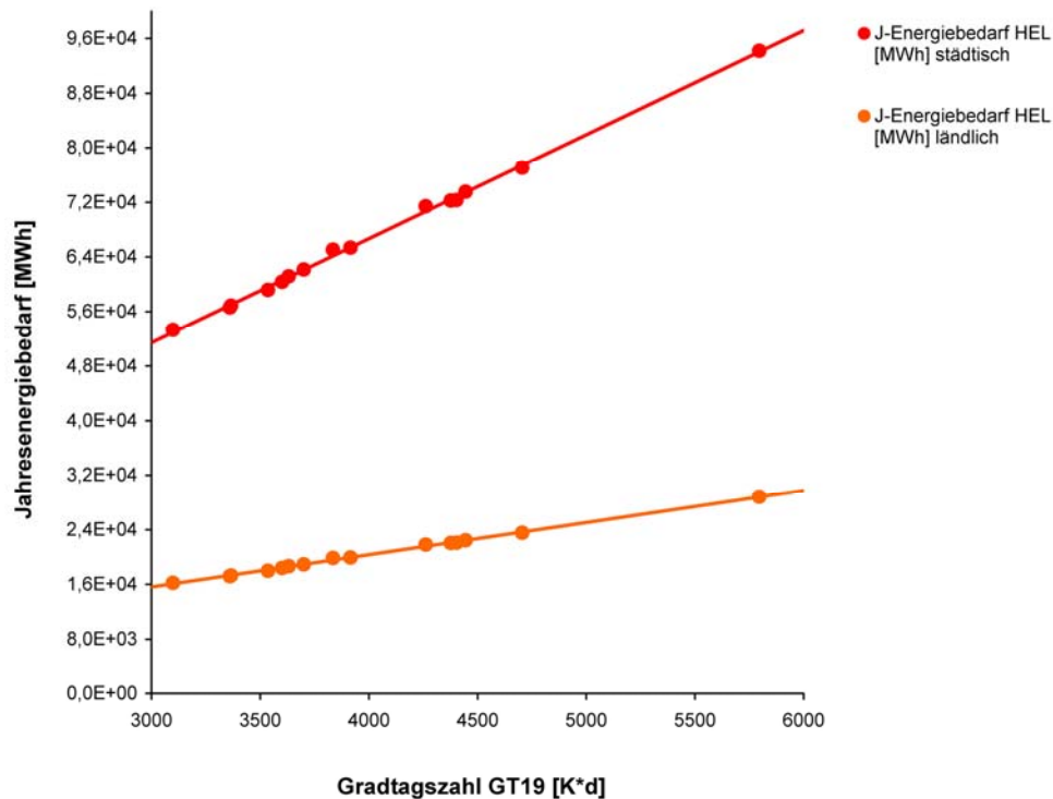
Bild 3-54 Jahresendenergiebedarf in Abhängigkeit der Gradtagszahl GT19 für das ländliche und städtische Gebiet, am Beispiel der Ölfeuerung (HEL: Heizöl EL)
