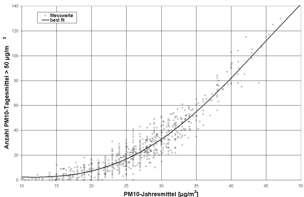
Bild 6-13 Anzahl der Tage mit mehr als 50 µg PM 10 /m 3 im Tagesmittel in Abhängigkeit vom PM 10 -Jahresmittelwert für Messstationen der Länder und des Umweltbundesamtes (1999-2003) sowie die daraus abgeleitete Funktion (BAST, 2005)
