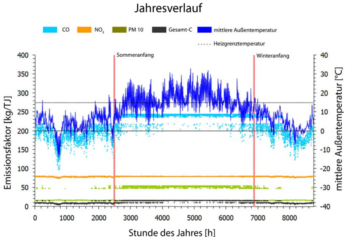
Bild 3-67 Jahresverläufe von Emissionsfaktoren für Pelletkessel im Nahwärmenetz für die Temperaturregion TRY 9
