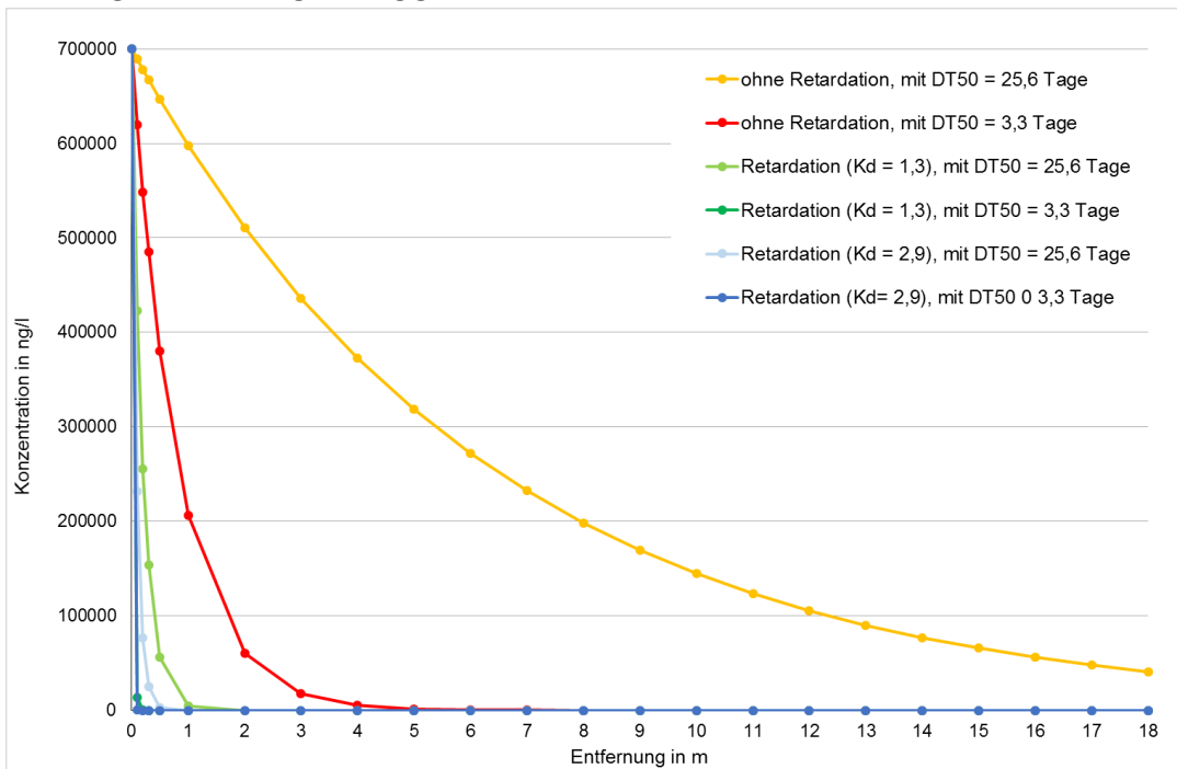
Abbildung 46: Entfernungsabhängiger Abbau von SMX im Grundwasser in Bösel
