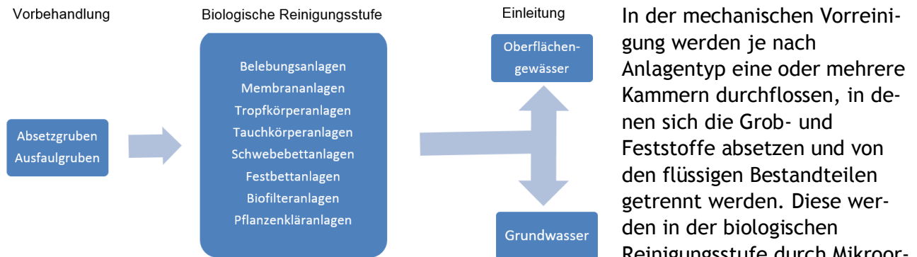
Abbildung 41: Übersicht über die KKA-Verfahrenssysteme (verändert nach 19 )
