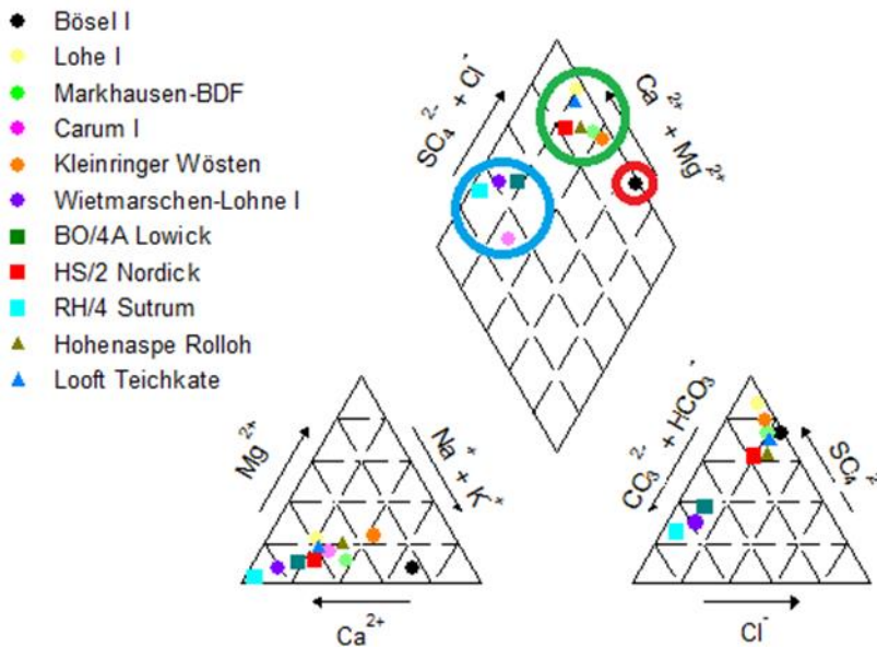
Abbildung 59: PIPER-Diagramm mit Analysen von 2012 bis 2015 und der Einteilung in Ca-SO 4 -(grüner Kreis), Ca-HCO 3 -(blauer) und Na-K-SO 4 -Typ (roter Kreis)
