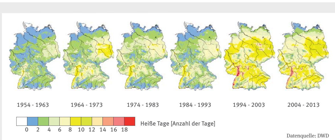
Abb. 6: Mittlere jährliche Anzahl der Heißen Tage mit einer Höchsttemperatur von mindestens 30 °C
