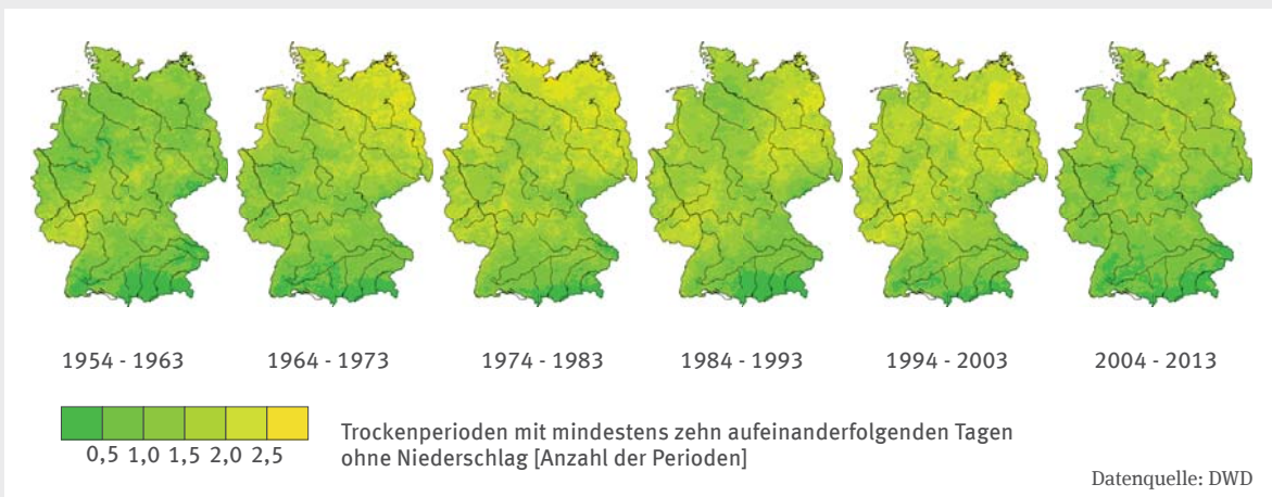
Abb. 12: Mittlere Anzahl von Trockenperioden mit mindestens zehn aufeinanderfolgenden Tagen ohne Niederschlag im meteorologischen Sommer
