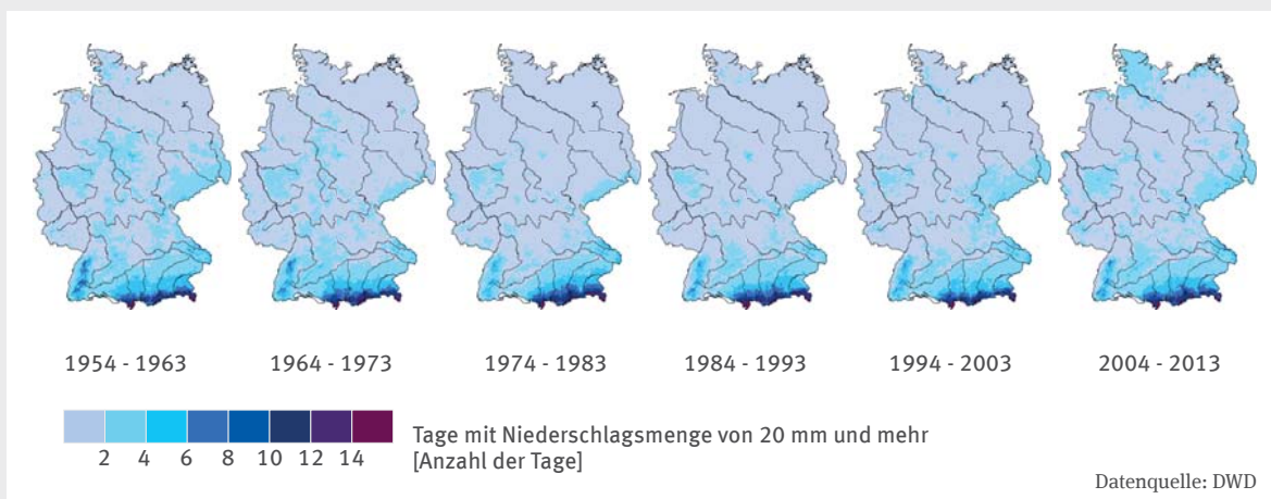
Abb. 10: Mittlere Anzahl der Tage mit einer Niederschlagsmenge von 20 mm und mehr im meteorologischen Sommer
